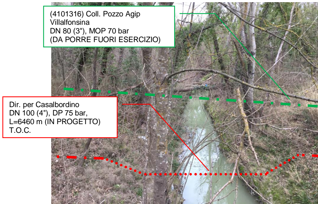
Foto n.5 – Vista Dir. per Casalbordino DN 100 (4") DP 75 bar, (IN PROGETTO) con attraversamento e metanodotto da porre fuori esercizio
