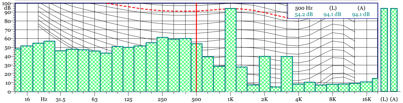
Esterne_.228 - 1/3 All Min Spectrum - Min
