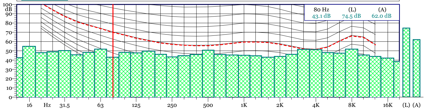
Esterne_.144 - 1/3 All Min Spectrum - Min
