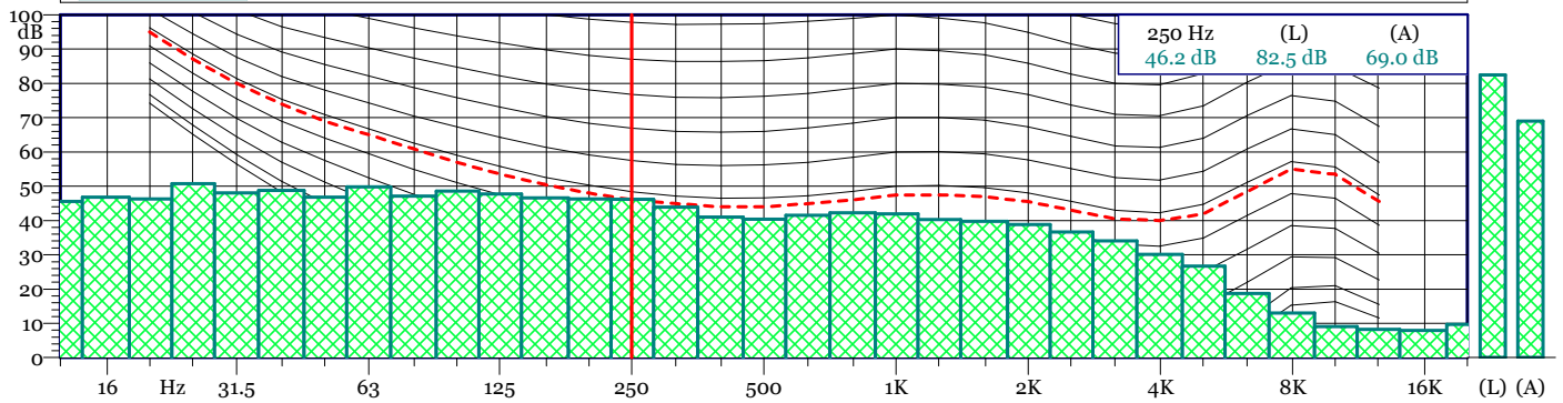
Esterne_.226 - 1/3 All Min Spectrum - Min
