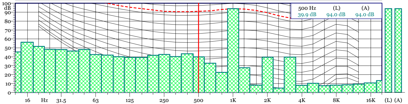
Esterne_.218 - 1/3 All Min Spectrum - Min
