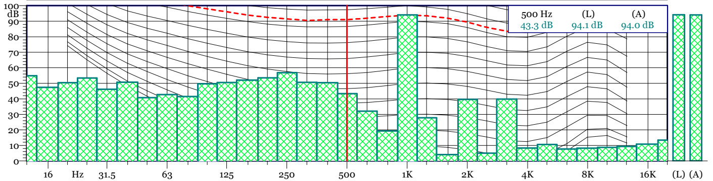
Esterne_.244 - 1/3 All Min Spectrum - Min
