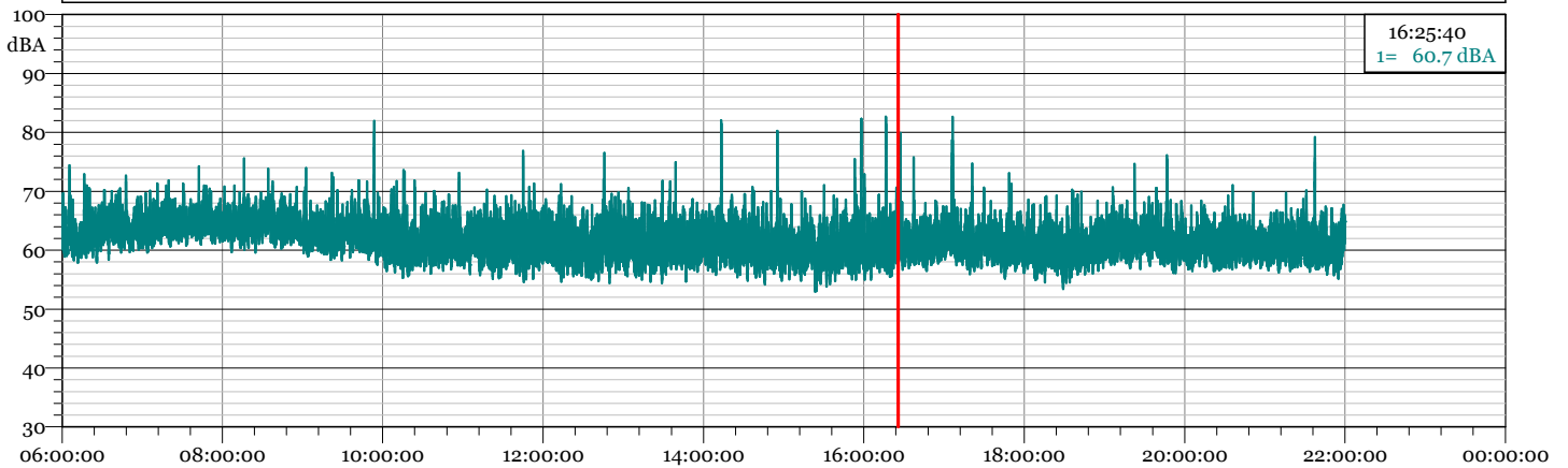
1 - TRD 19121200.LD0 - 1/3 Leq Spectrum + SLM - LAeq
