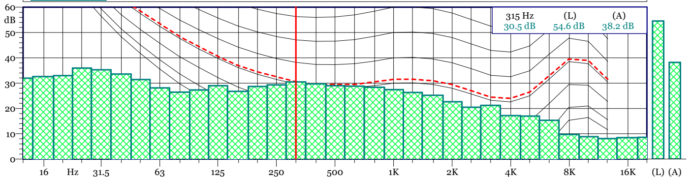
P16 TRD.LD0 1/3 All Min Spectrum - Min
