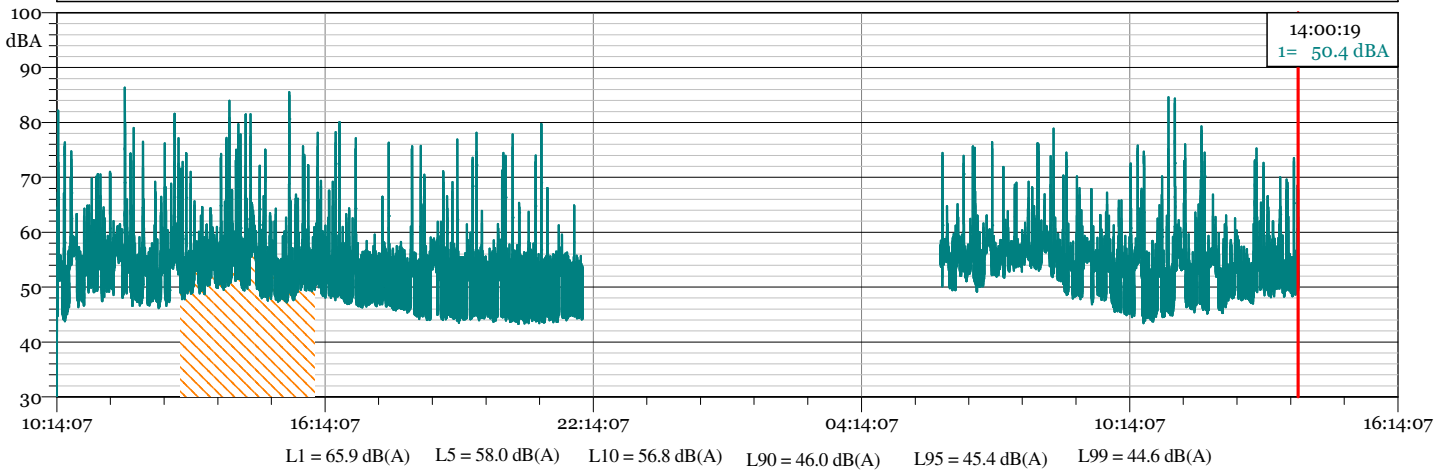
P15 TRD.LD0 1/3 Leq Spectrum + SLM - LAeq
