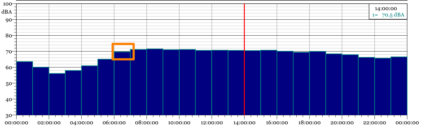
1 - Intervalli -19121100.LDO - Leq - LAeq
