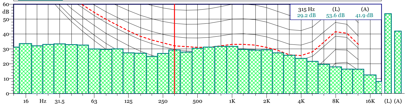
P15 TRD.LD0 1/3 All Min Spectrum - Min
