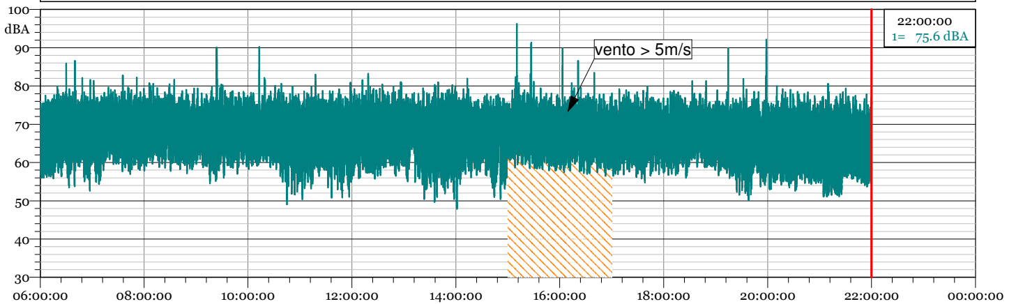
1 - TRD 19121200.LDo - 1/3 Leq Spectrum + SLM - LAeq
