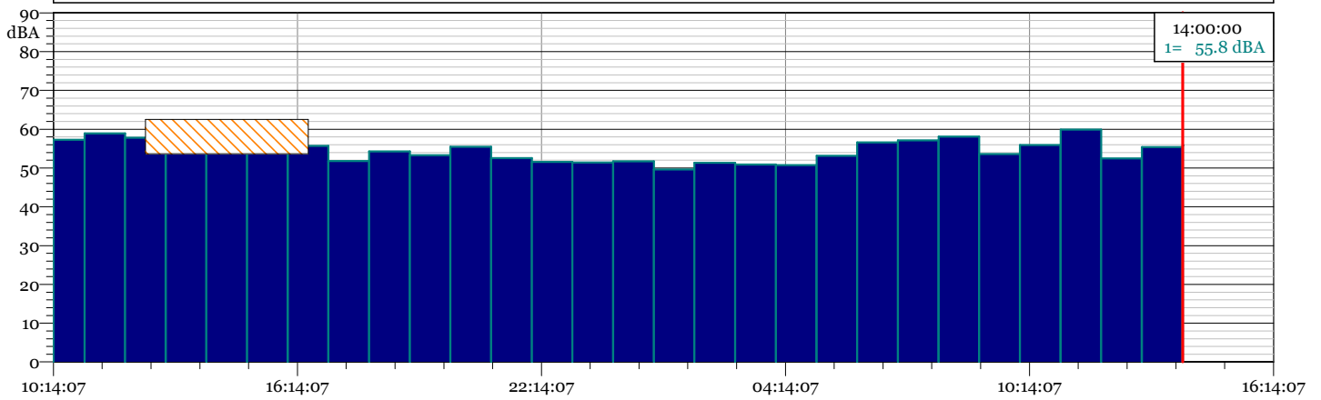
1 - Intervalli - P15 TOT.LD0 - Intervals - Leq
