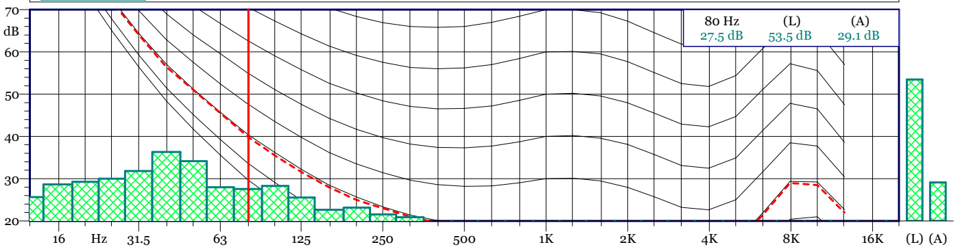
P20 TOT.LDo 1/3 All Min Spectrum - Min
