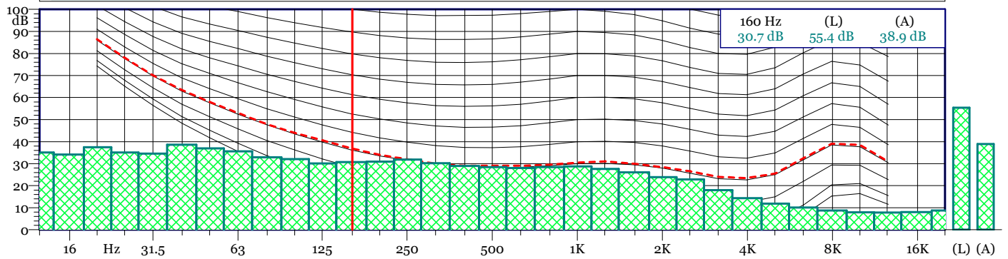
Esterne_.216 - 1/3 All Min Spectrum - Min
