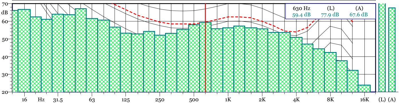
P16 TRN.LD0 Intv 1/3 Max Spectrum - Min
