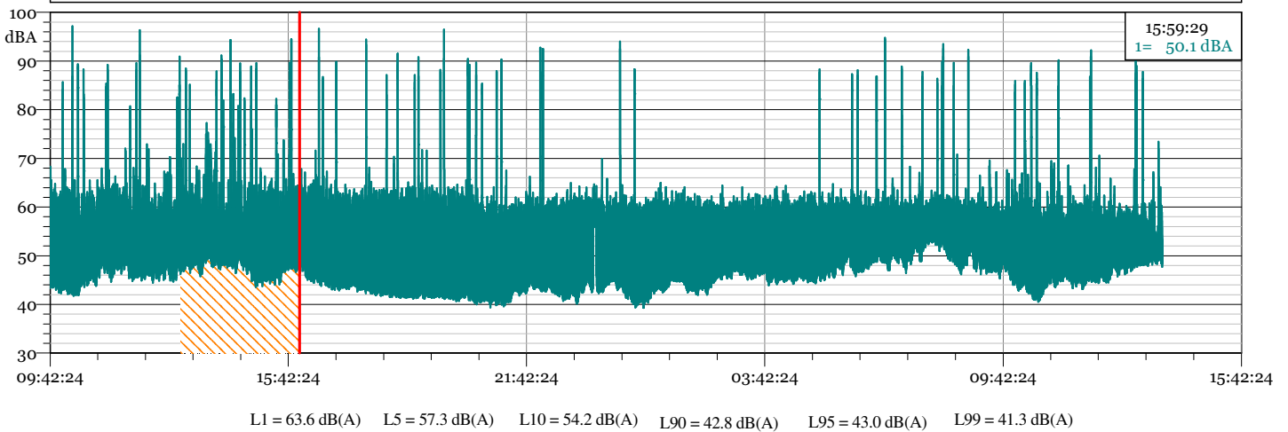
P16 TOT.LDo 1/3 Leq Spectrum + SLM - LAeq
