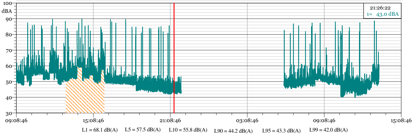
P20 TRD.LD0 1/3 Leq Spectrum + SLM - LAeq
