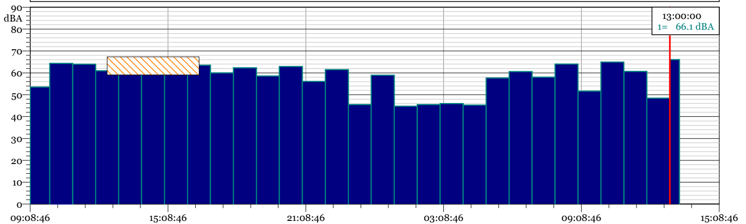
1 - Intervalli -P20 TOT.LDO - Intervals - Leq
