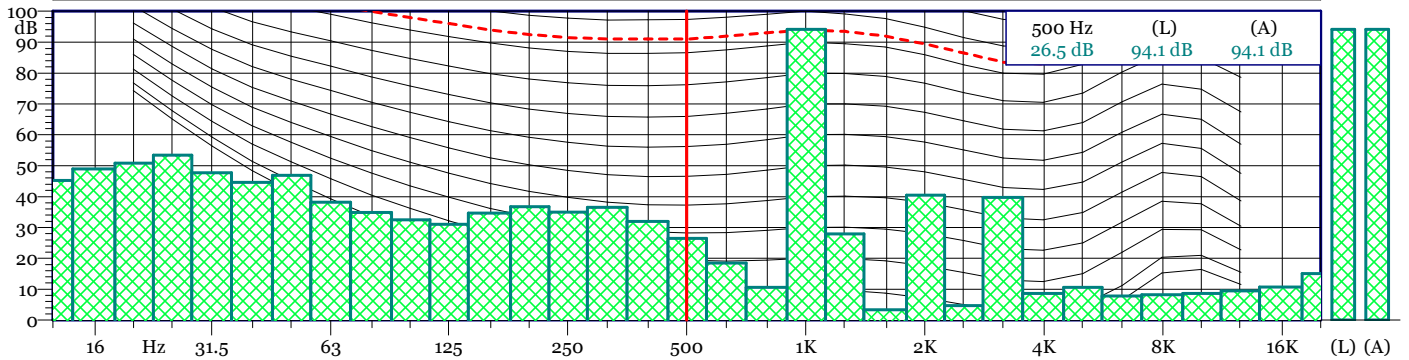
Esterne_.197 - 1/3 All Min Spectrum - Min
