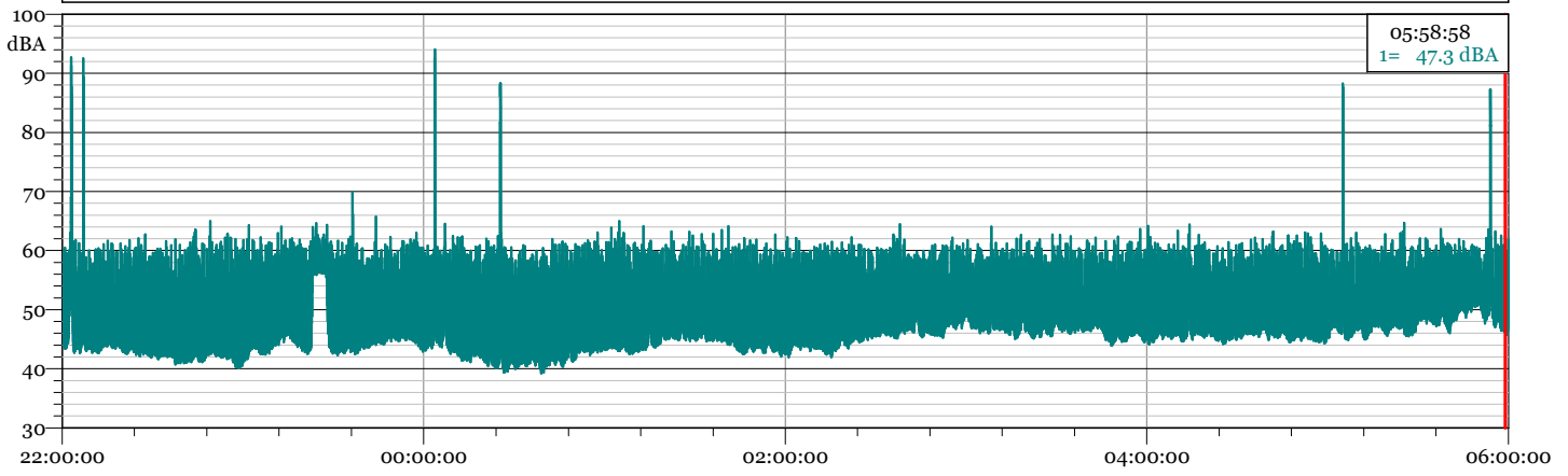
P16 TRN.LD0 1/3 Leq Spectrum + SLM - LAeq
