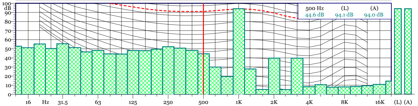
Esterne_.235 - 1/3 All Min Spectrum - Min
