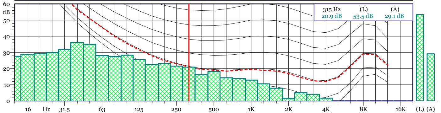
P20 TRD.LD0 1/3 All Min Spectrum - Min
