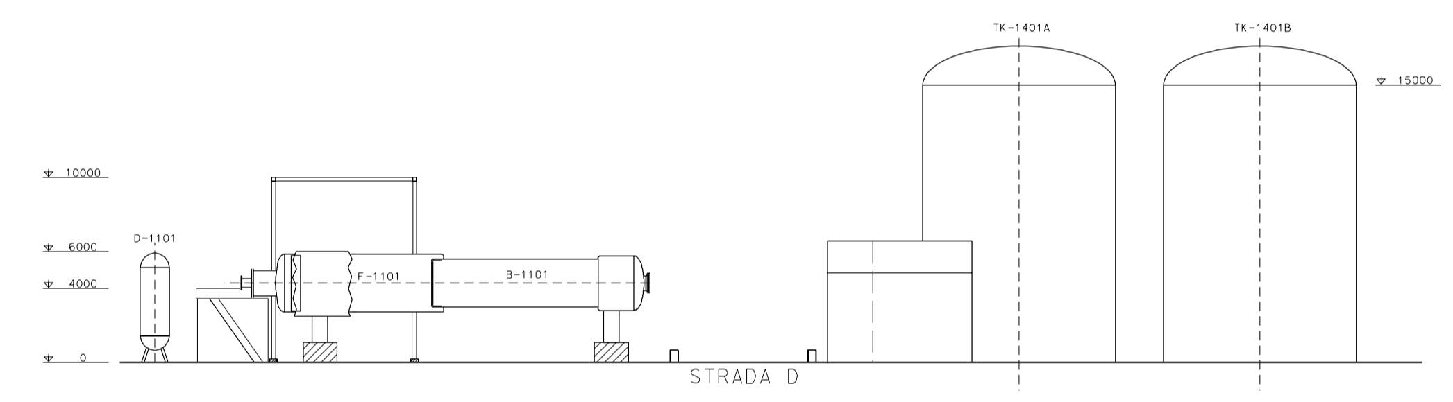
SEZIONE B-B
