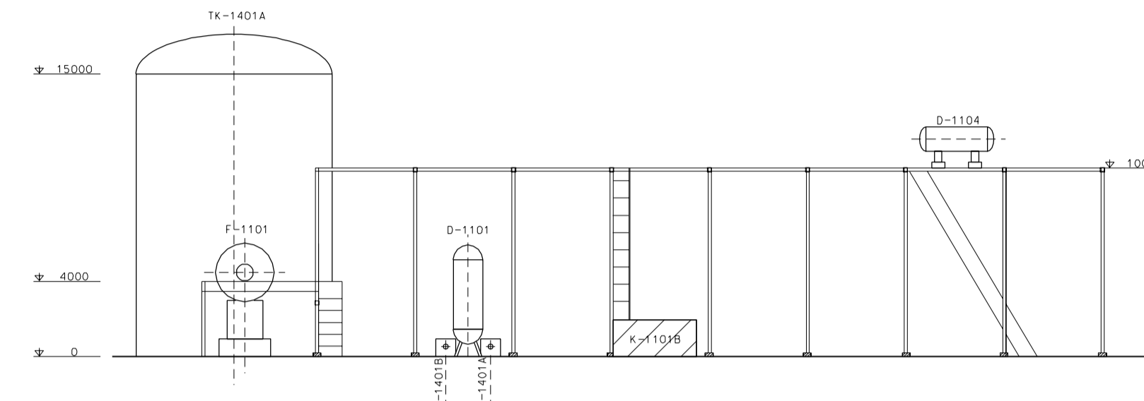
SEZIONE A-A
