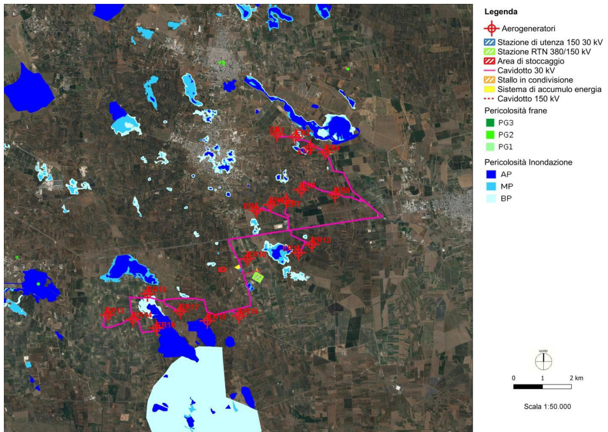
Figura 3 - Inquadramento su Carta di Pericolosità Idraulica
