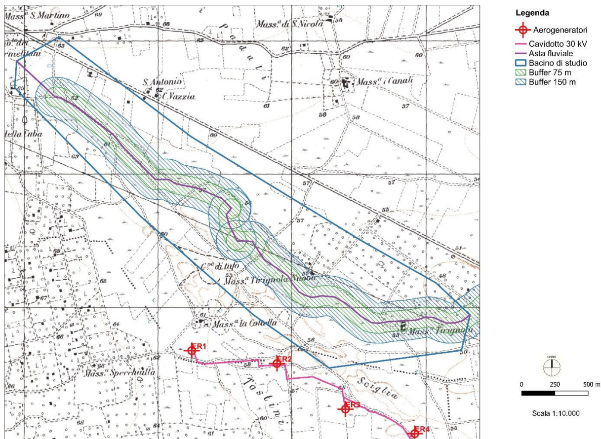
Figura 6 - Individuazione bacino di studio su base IGM
