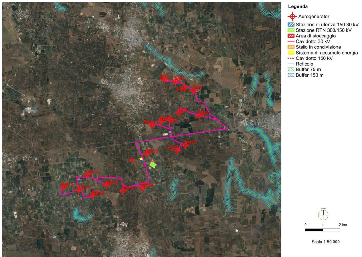
Figura 5 - Area di intervento con buffer di 150 metri del reticolo
