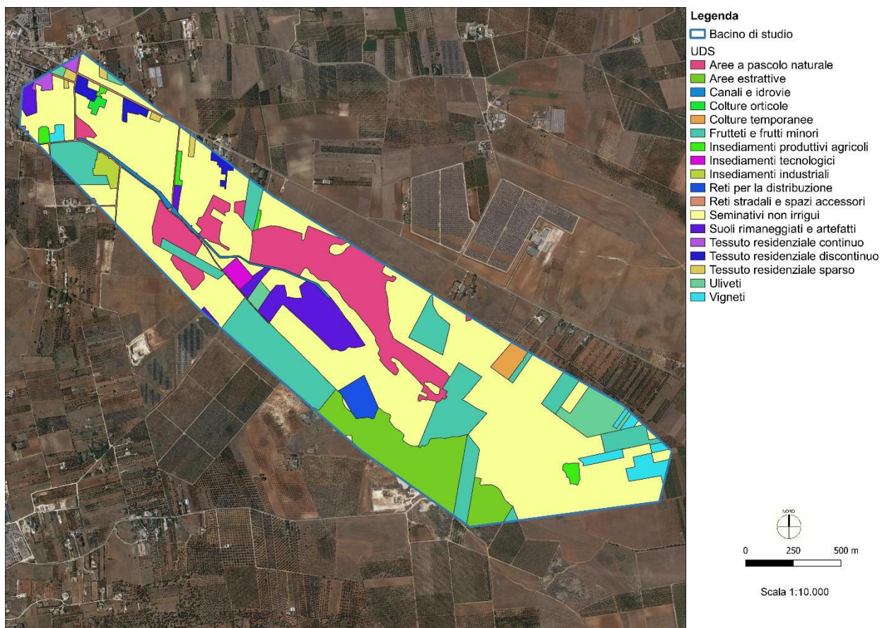
Figura 9 - Sovrapposizione bacino con Uso Del Suolo
