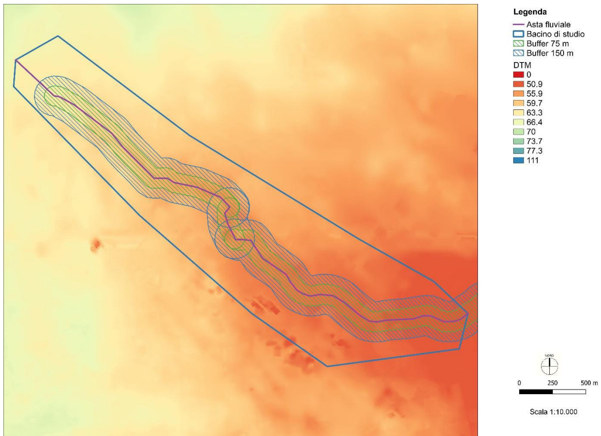
Figura 8 - Individuazione del bacino di studio su base D.T.M.
