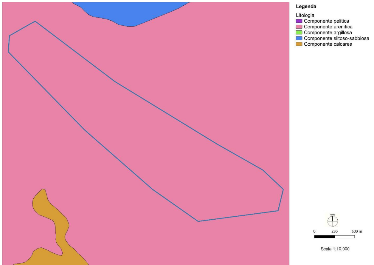
Figura 10 -Sovrapposizione bacino con Carta Litologica
