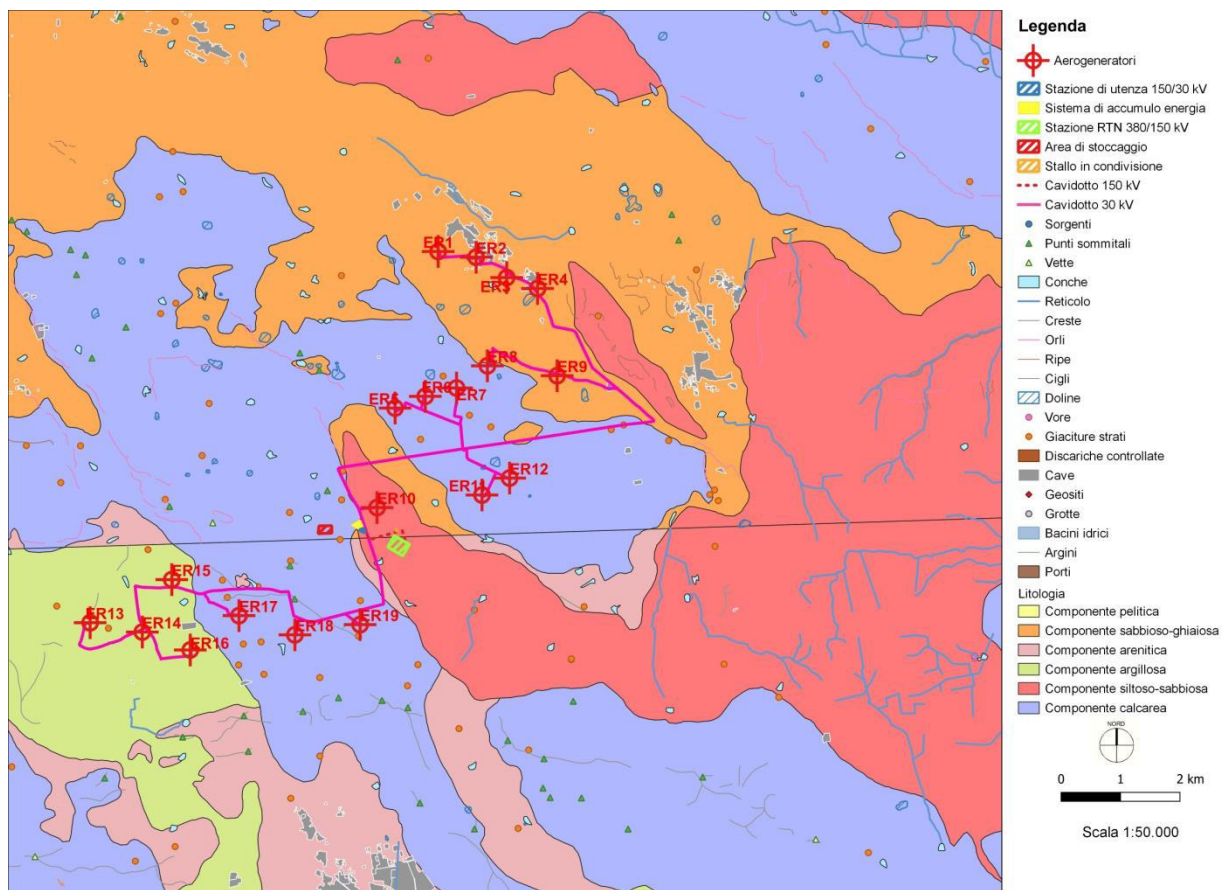
Figura 4 - Area d'intervento su Carta Idrogeomorfologica
