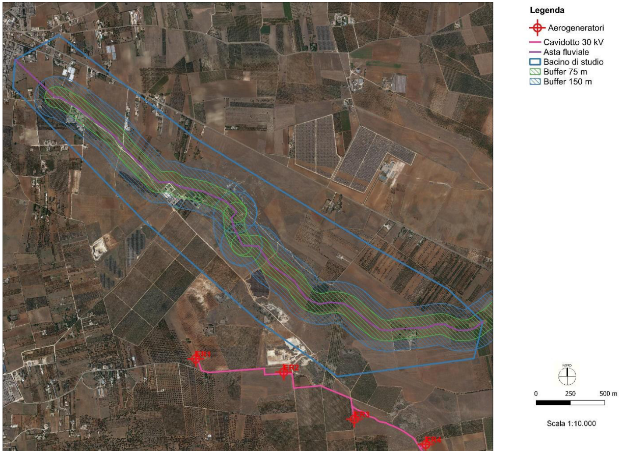
Figura 7 - Individuazione bacino di studio su ortofoto
