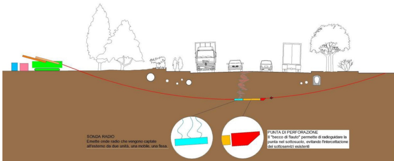
Fase 1: Realizzazione foro pilota con controllo altimetrico
