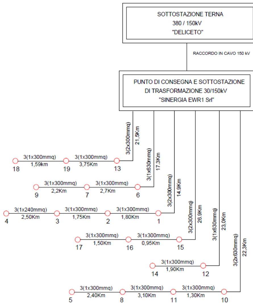
Schema elettrico unifilare WTG
