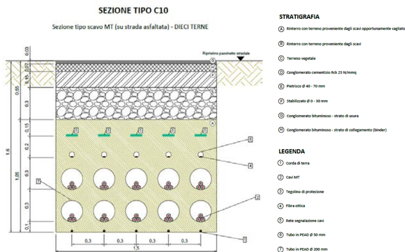
Sezioni tipo cavidotto tipo C
