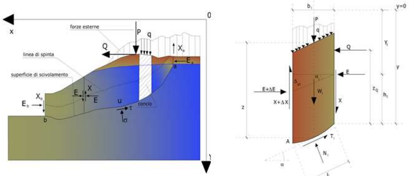
Azioni sul cuneo i -esimo secondo le ipotesi di Janbu e rappresentazione d'insieme dell'ammasso
