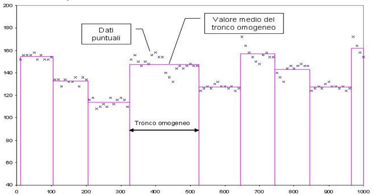
Figura 2 – Diagramma individuazione "tronchi omogenei"
