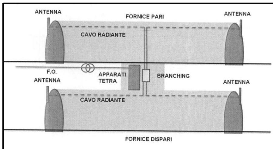
Tipologico installazione sistema TETRA per gallerie a doppio fornice
