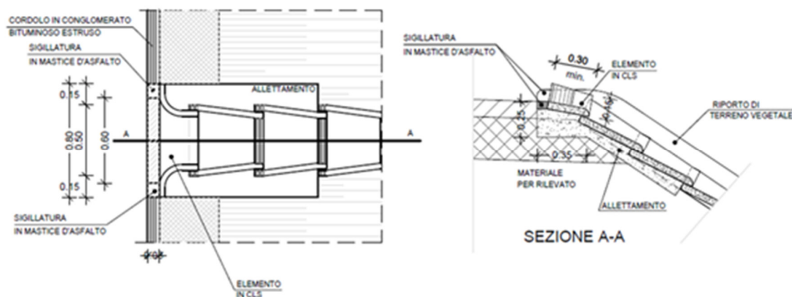
Figura 8.2 - Embrice tipo.
