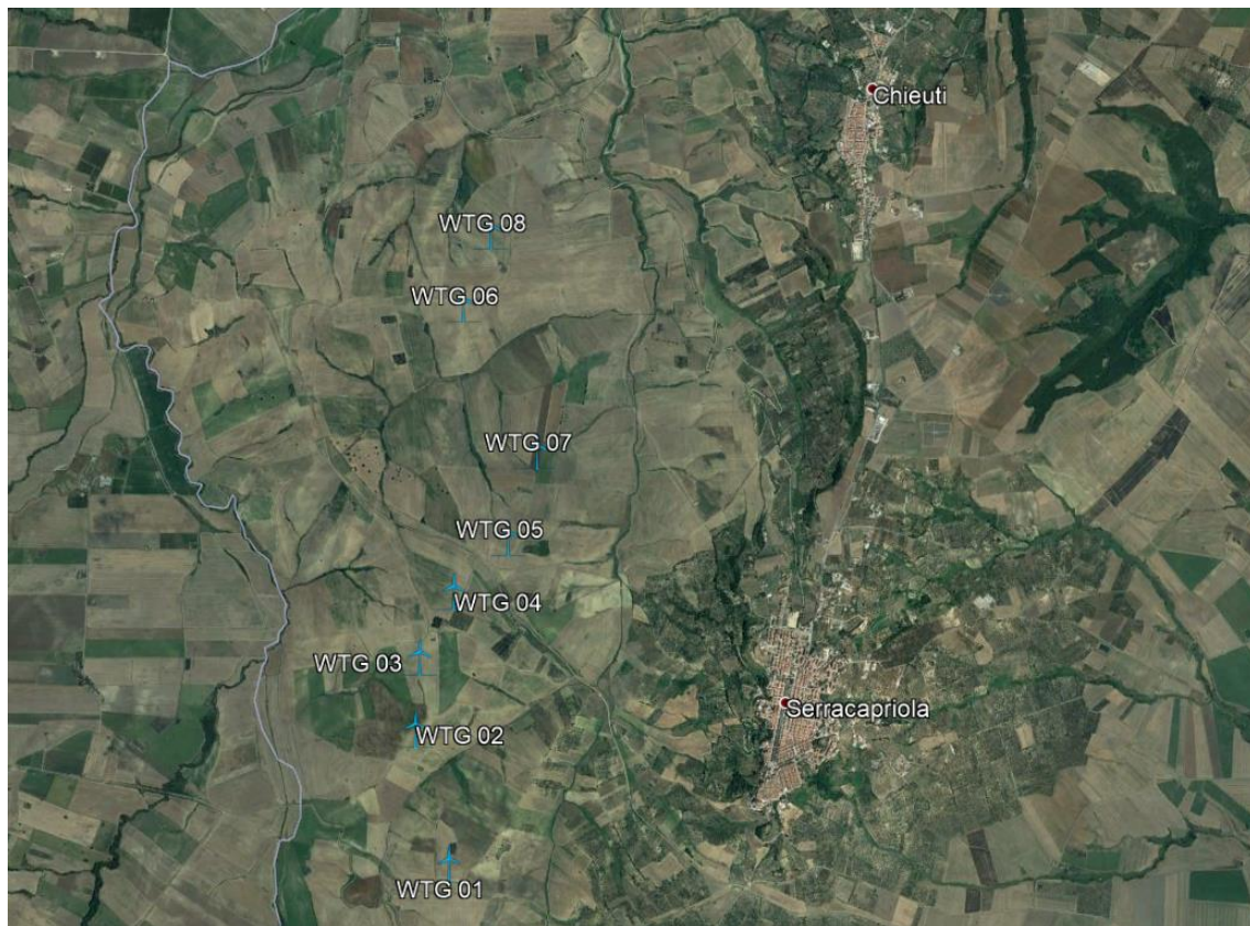
Figura 1 - Individuazione su ortofoto dell'impianto in progetto
