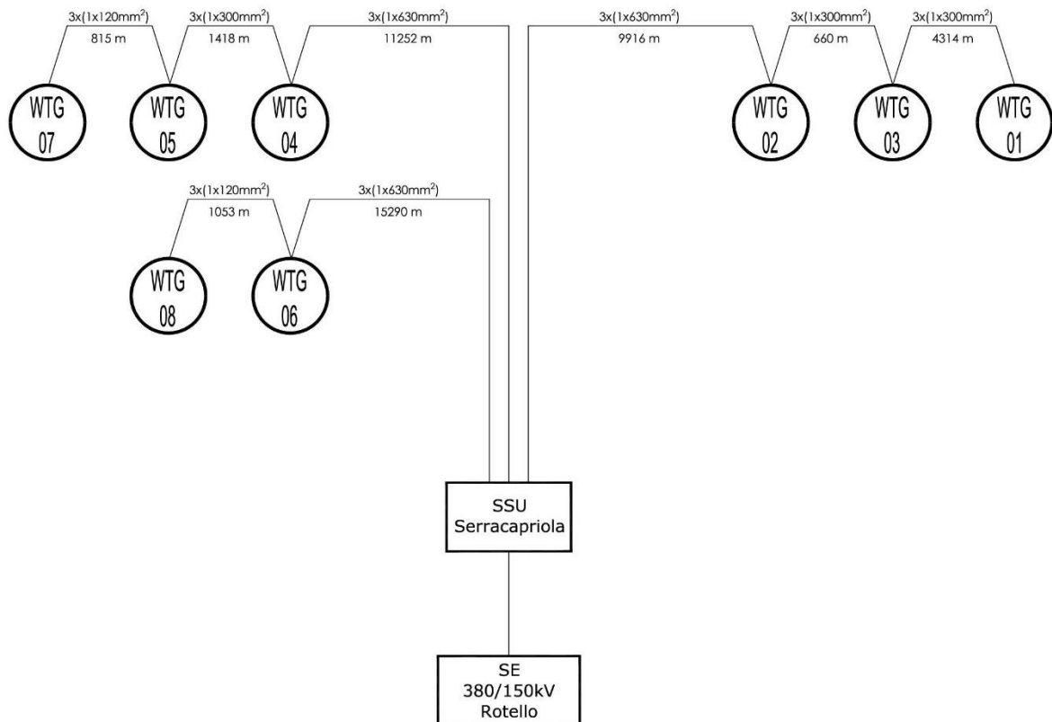
Figura 3 – Schema a blocchi della Wind Farm
