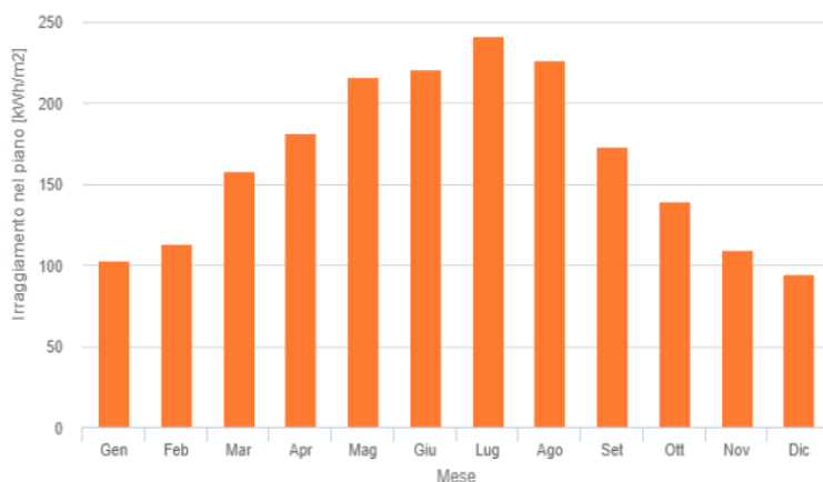
Figura 2 – Media Mensili di irraggiamento al metro quadrato sui moduli del sistema scelto (Fonte PVGIS – SARAH)
