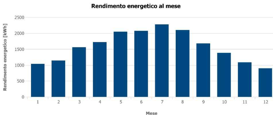
Figura 4 – Rendimento energetico mensile del Generatore FV
