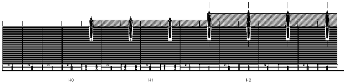
Sezioni-tipo dei moduli di barriera antirumore previsti nello Studio Acustico
