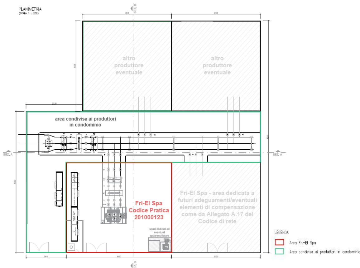
Figura 2: schema architettonico della SET
