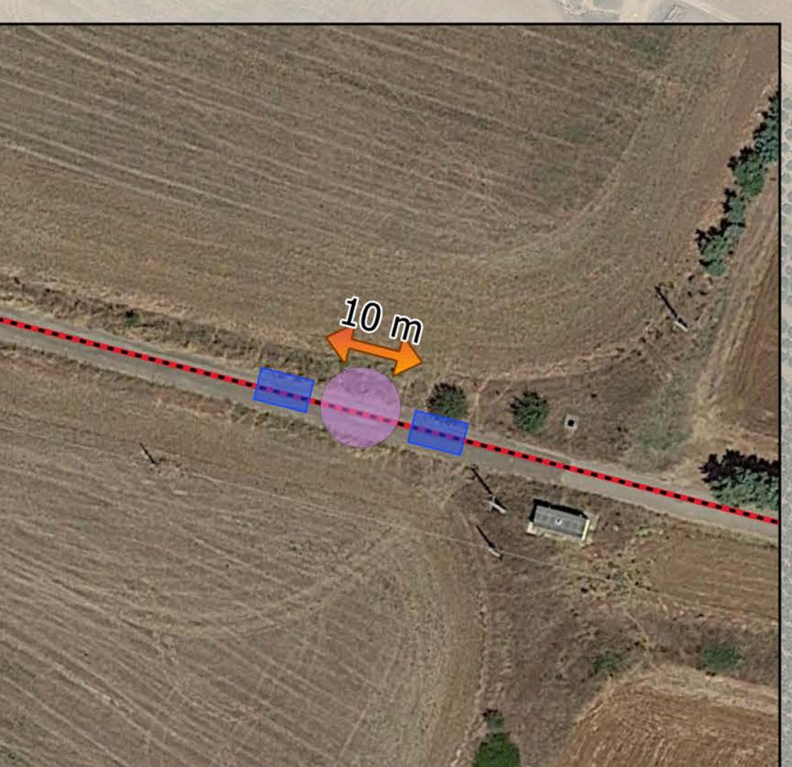
DETTAGLIO INTERFERENZA N. 7 Scala 1 : 500
