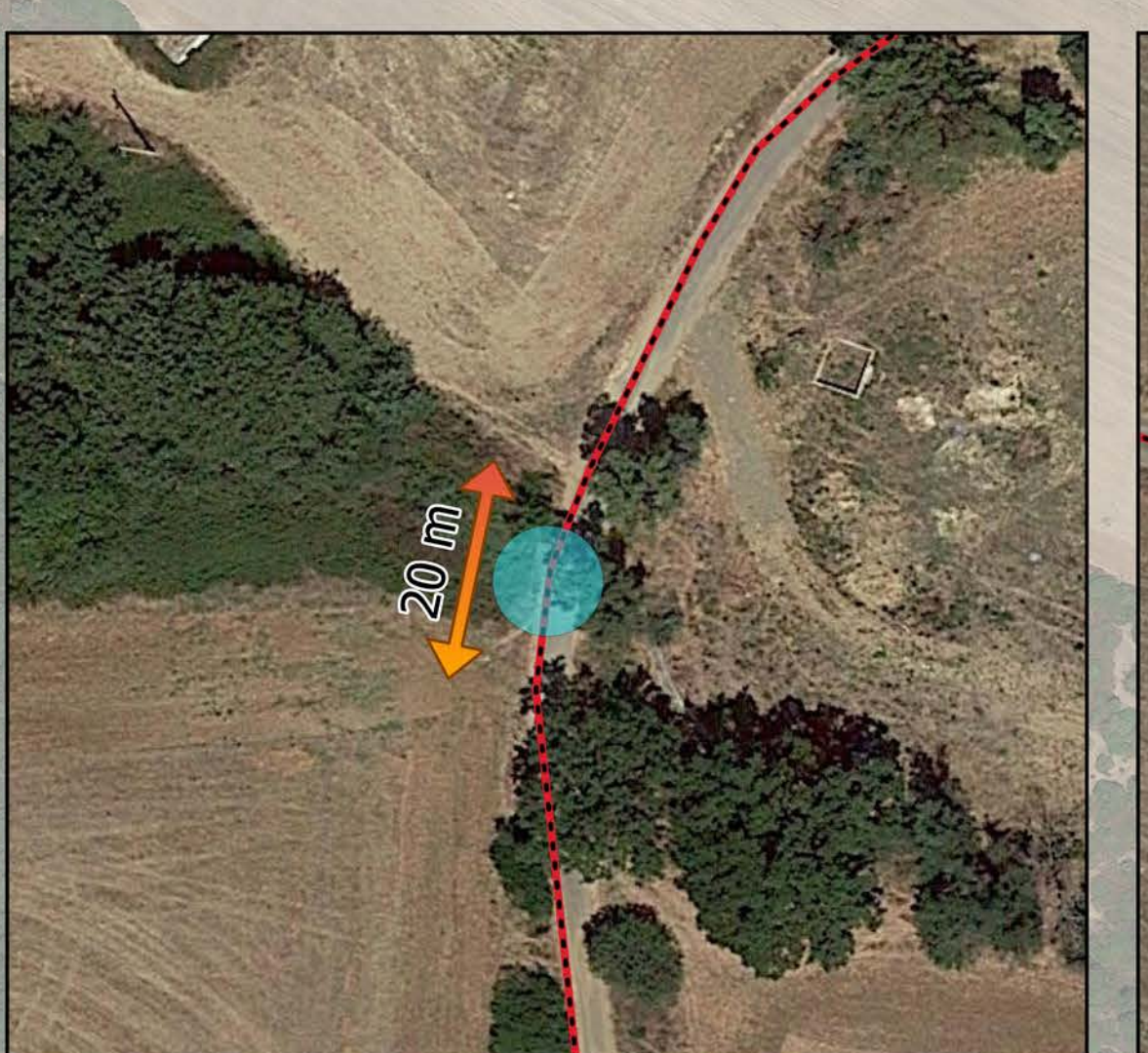
DETTAGLIO INTERFERENZA N. 6 Scala 1 : 500
