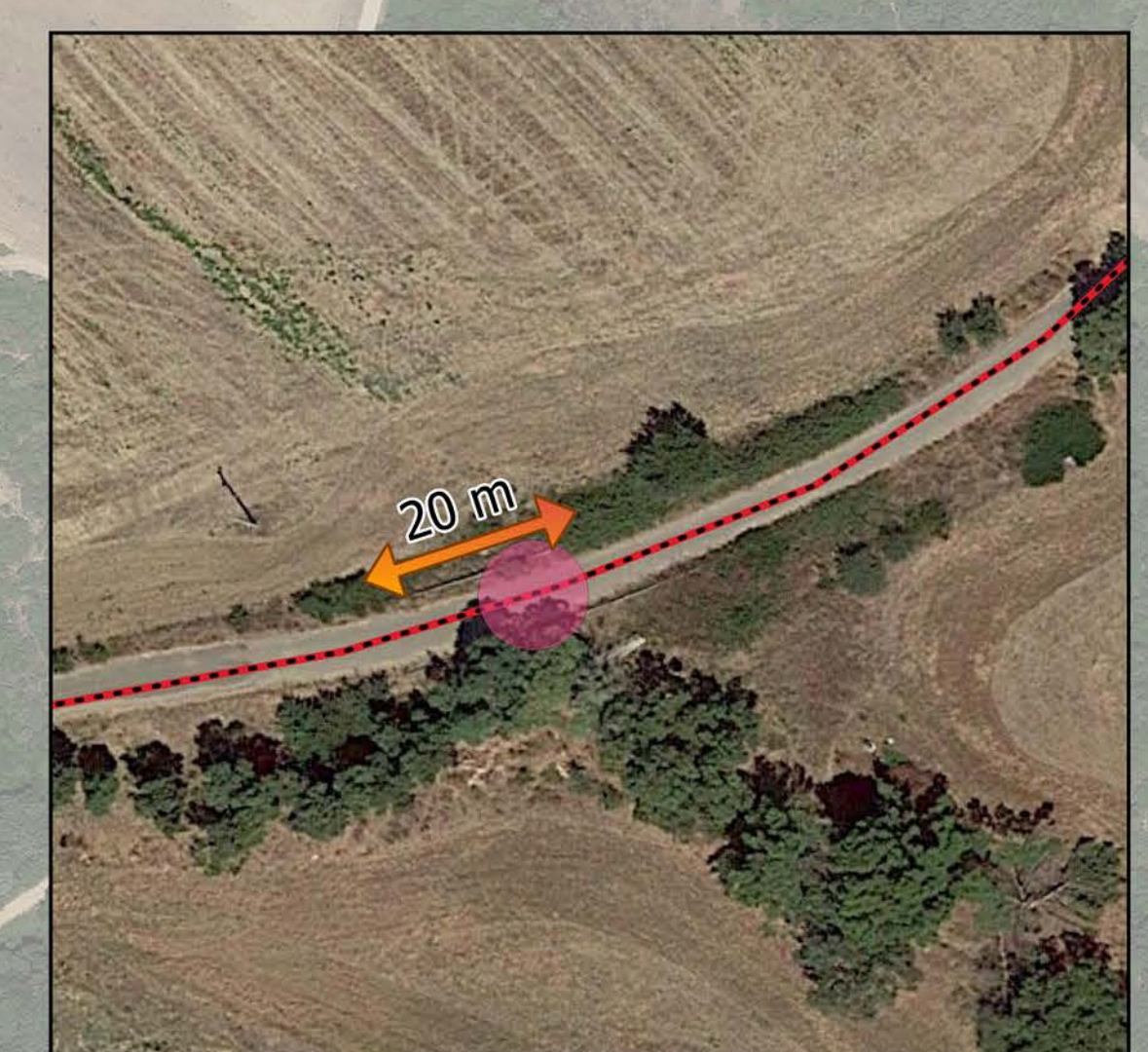
DETTAGLIO INTERFERENZA N. 5 Scala 1 : 500
