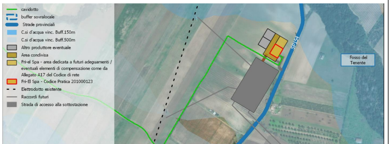
Figura 3: Sovrapposizione di parti del cavidotto e della sottostazione con il buffer dei corsi d'acqua vincolati
