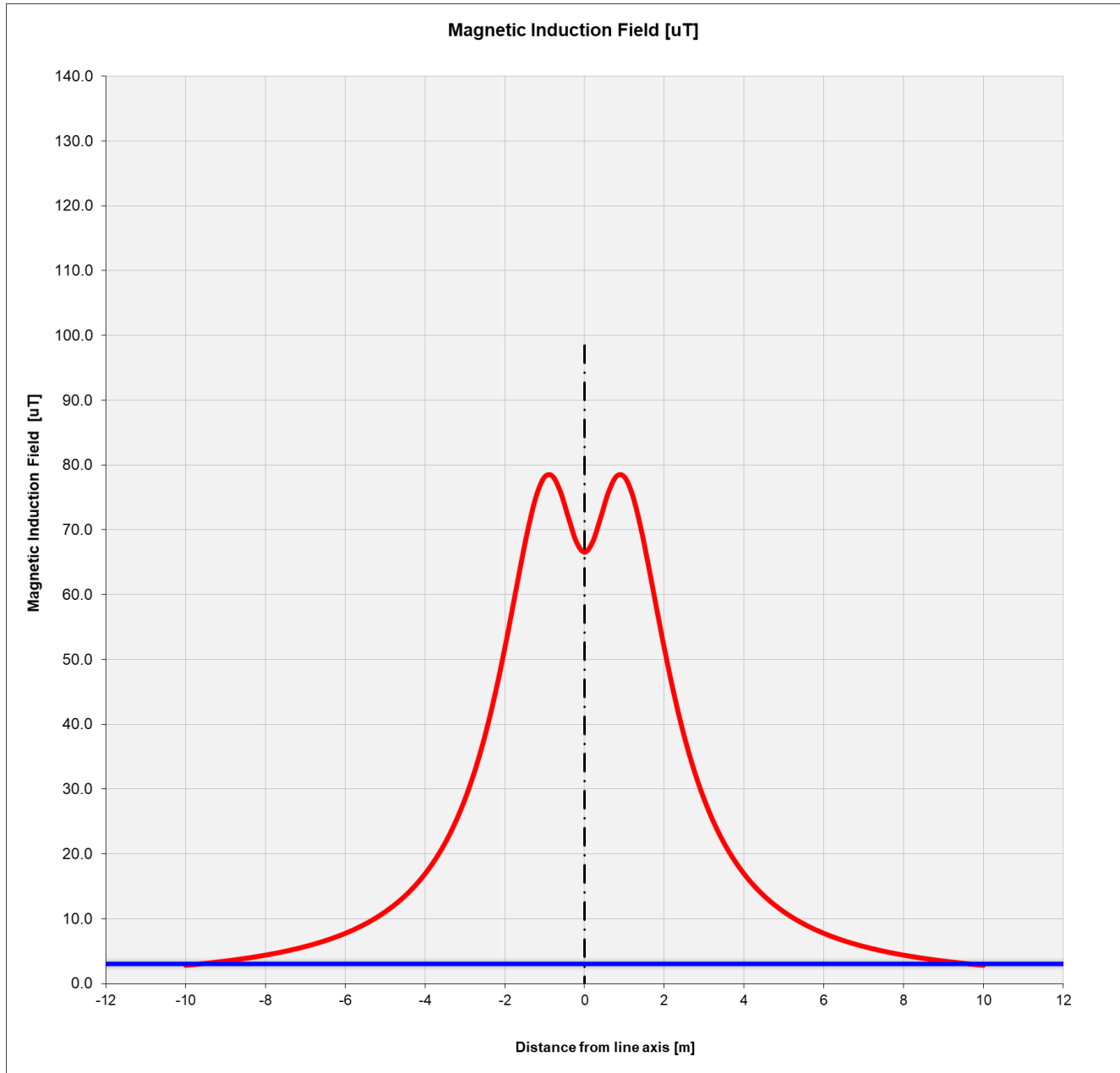
Figura 32: Andamento dell'induzione magnetica prodotta dalla linea in cavo AT (posa in piano e terna doppia)
