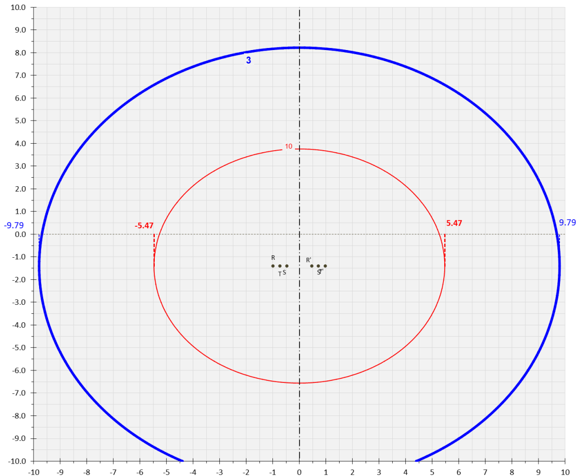
Figura 53: Isolinee dell'induzione magnetica nel caso del cavo interrato da 2500 mm 2 (doppia terna)
