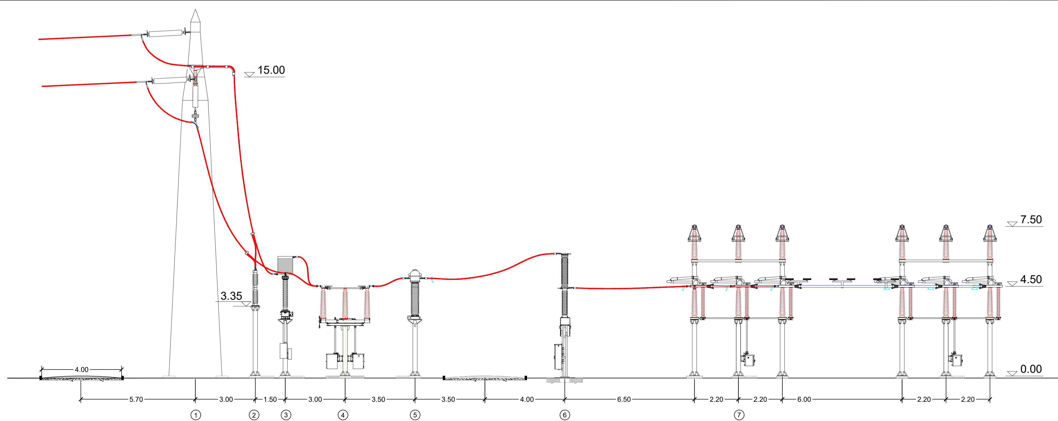
SEZIONE AA' - STALLO DI ARRIVO IN STAZIONE TERNA
