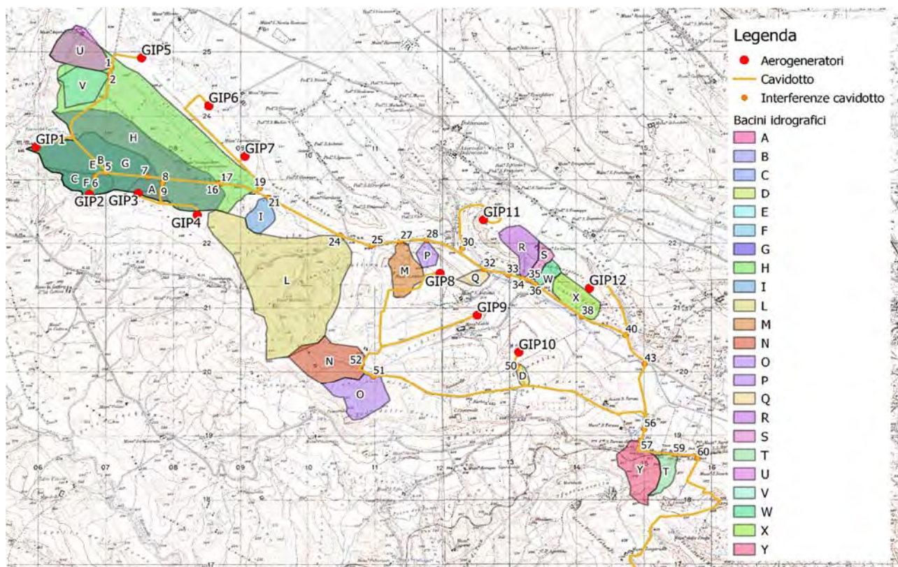
Figura 4. Interferenze tra il reticolo idrografico e le opere in progetto
