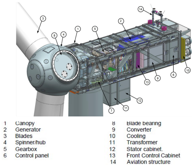
Figura 2 : Schema aerogeneratore
