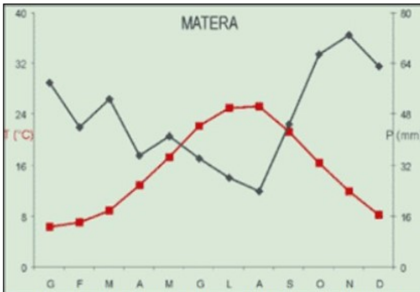
Figura - Diagramma bioclimatico di Bagnouls & Gausson relativo alla stazione termopluviometrica di Matera (Fonte: www.basilicatanet.it ).
