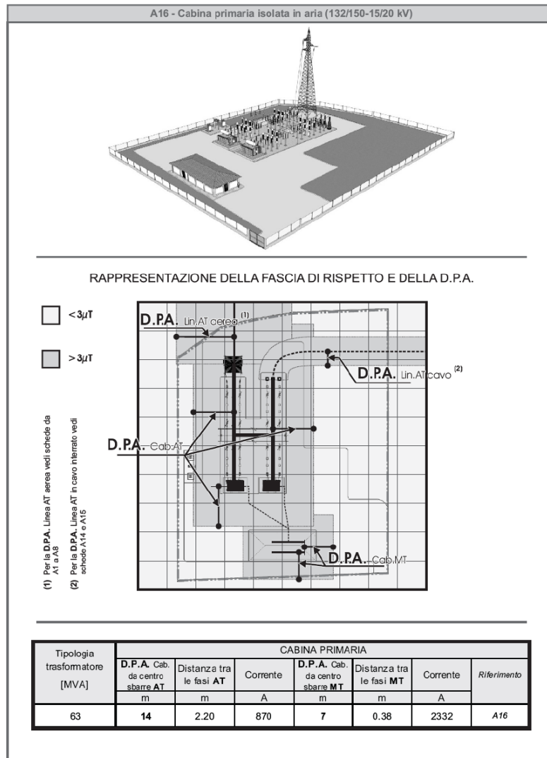
Figura 7 - Esempio di fasce di rispetto relative ad una cabina primaria
