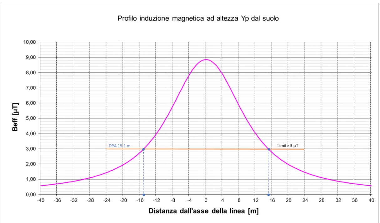
Figura 9: Andamento del campo magnetico in funzione della distanza dall'asse dei conduttori in forma grafica relativa all'elettrodotto aereo AT ad un'altezza di 1,5 m dal suolo (il valore del campo magnetico è in scala decimale)
