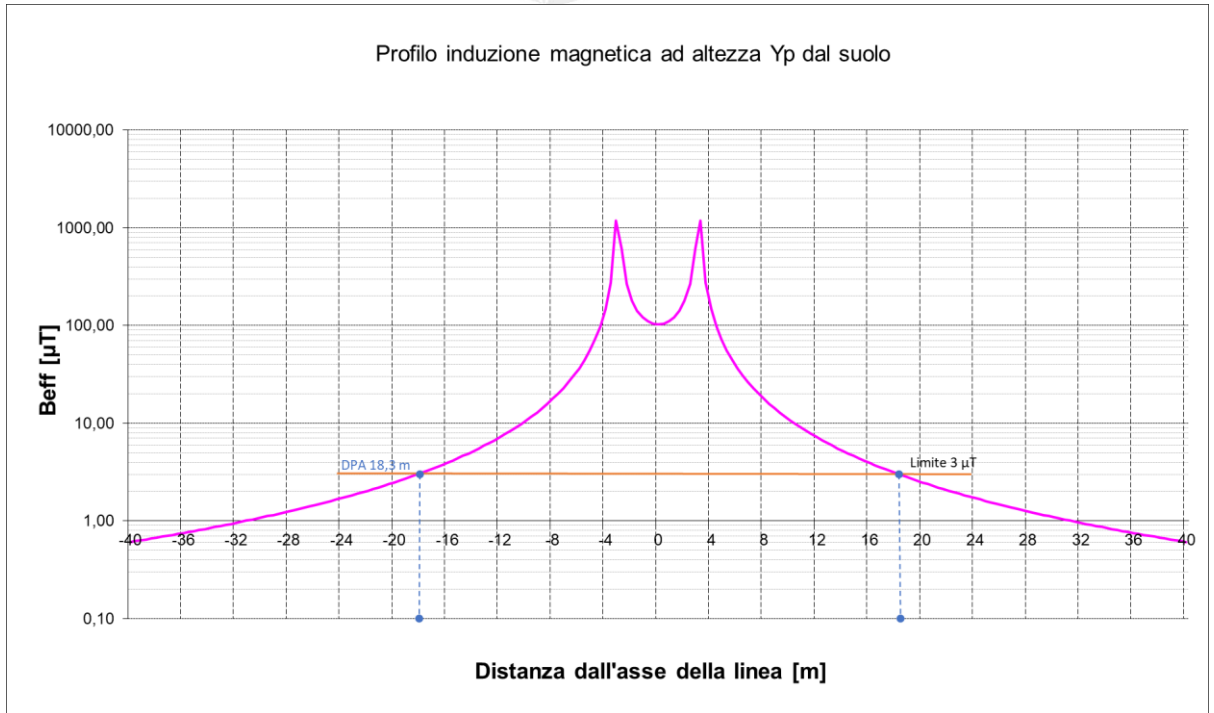
Figura 8: Andamento del campo magnetico in funzione della distanza dall'asse dei conduttori in forma grafica relativa all'elettrodotto aereo AT all'altezza dei conduttori (il valore del campo magnetico è in scala logaritmica)
