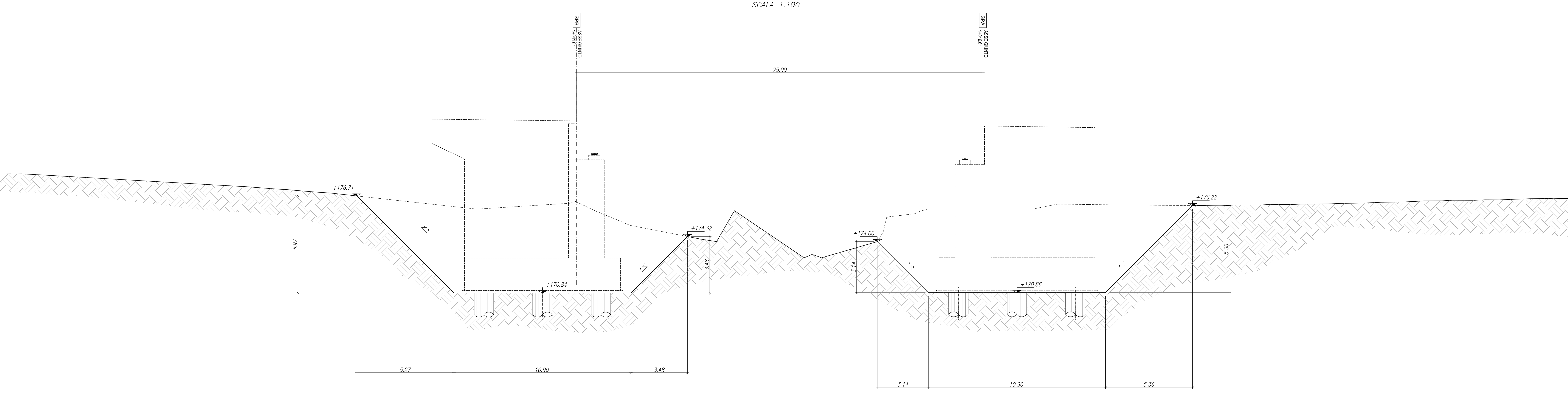
PONTE STRADALE IV04 SEZIONE LONGITUDINALE SCALA 1:100
