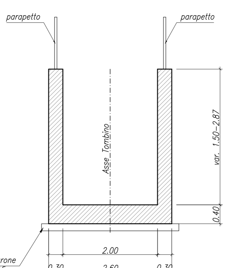
TOMBINO STRADALE IN21 SEZIONE C-C SCALA 1:50
