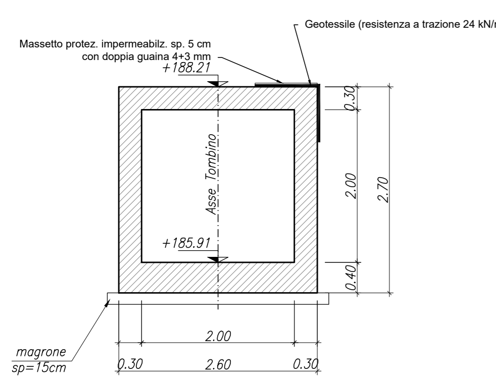
TOMBINO STRADALE IN21 SEZIONE A-A SCALA 1:50
