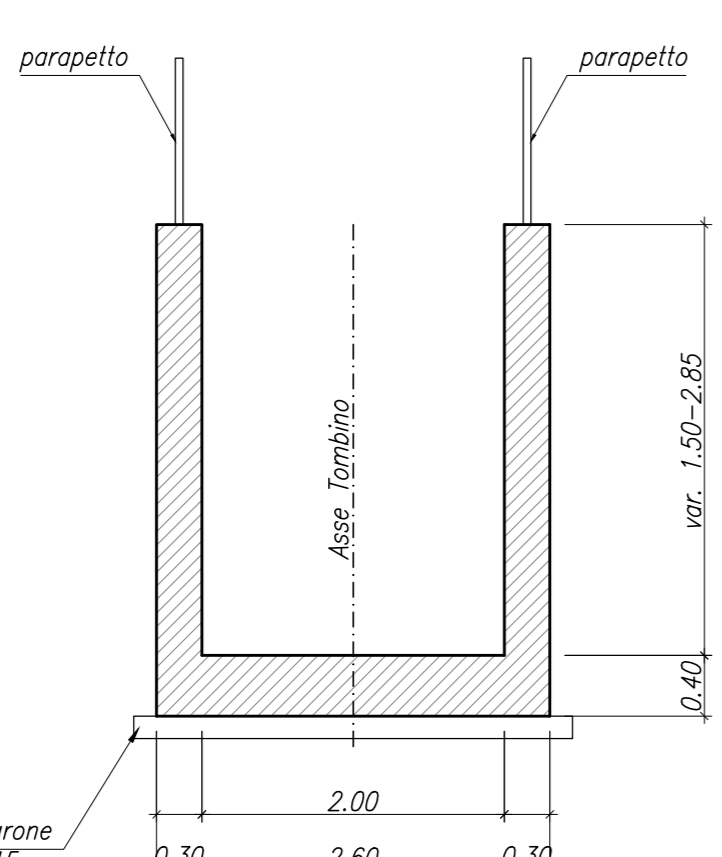
TOMBINO STRADALE IN21 SEZIONE B-B SCALA 1:50
