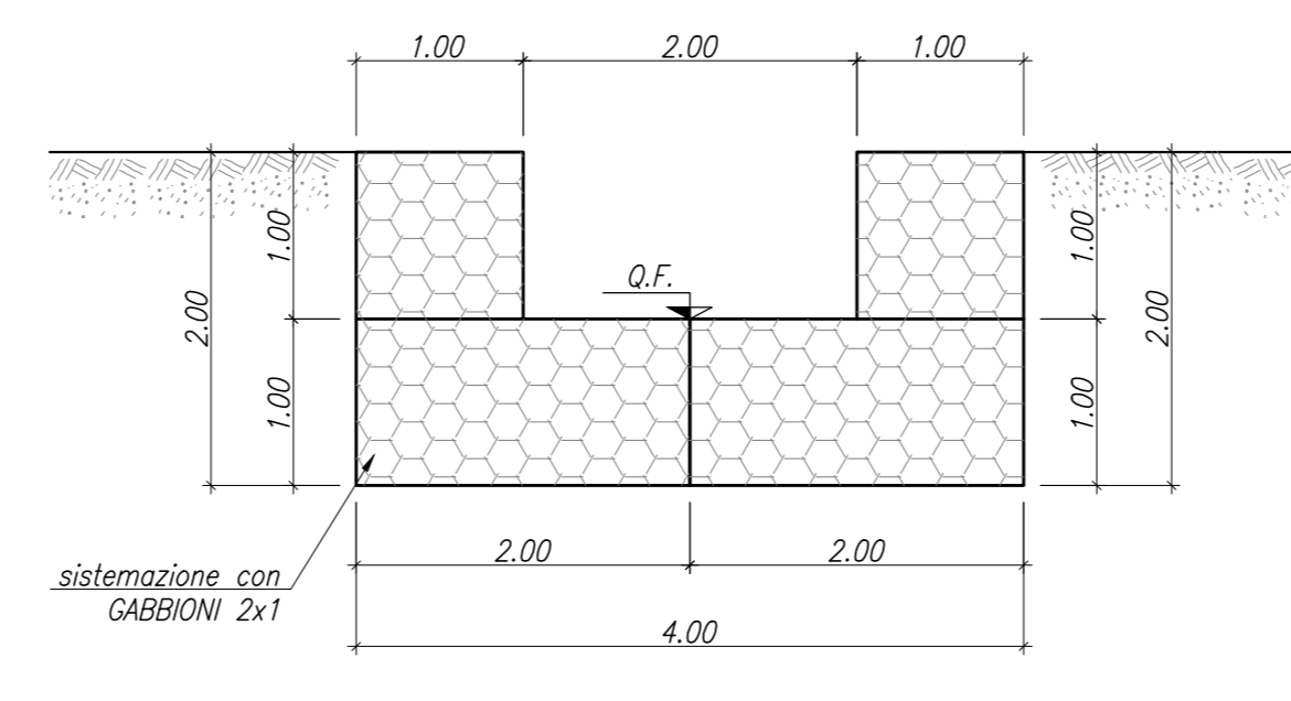
TOMBINO STRADALE IN21 SEZIONE TIPO GABBIONE 2x1 SCALA 1:50
