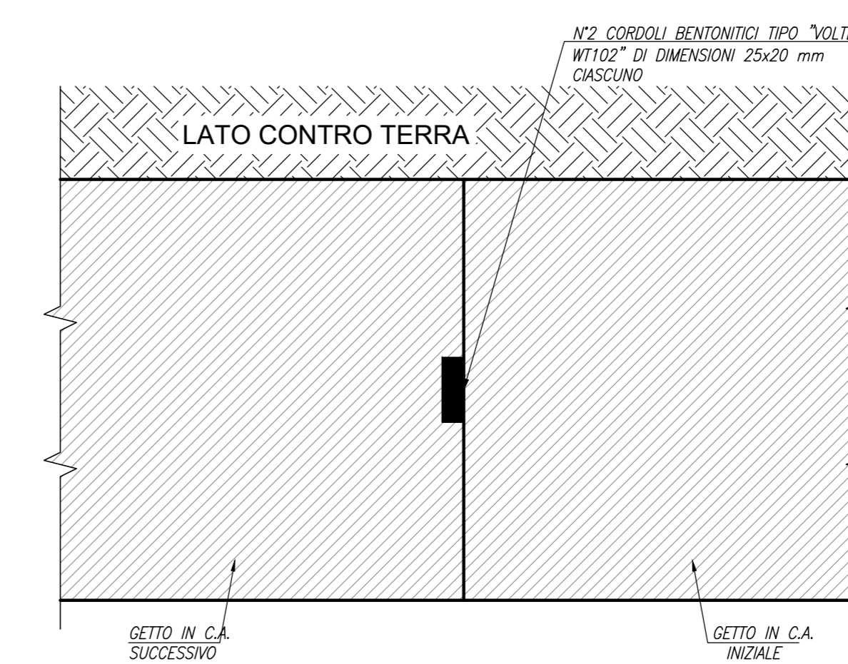
PARTICOLARE GIUNTO STRUTTURALE CORDONE BENTONITICO SCALA 1:10
