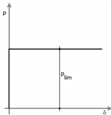
Comportamento palo-terreno
