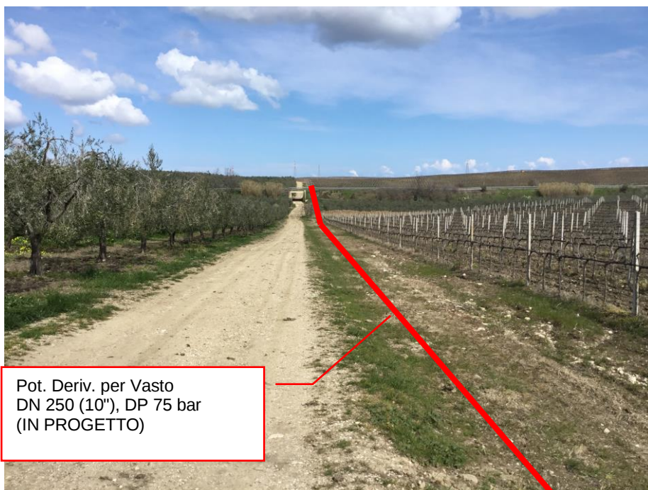
Foto n.6 – Km 1+140 - Panoramica Pot. Der. per Vasto DN 250 (10'') DP 75 bar (IN PROGETTO)
