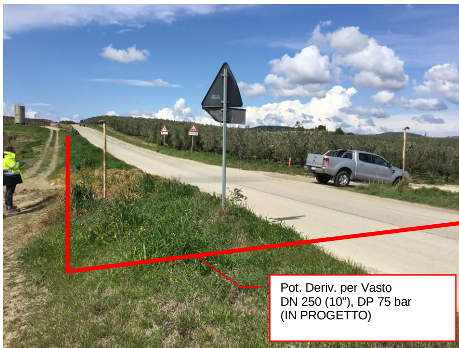
Foto n.5 – Km 1+025 - Vista su strada del Pot. Der. per Vasto DN 250 (10'') DP 75 bar (IN PROGETTO)
