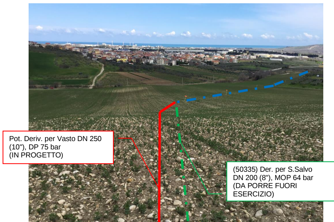
Foto n.10 – Km 3+000 - Panoramica metanodotti da porre fuori esercizio, esistente e in progetto
