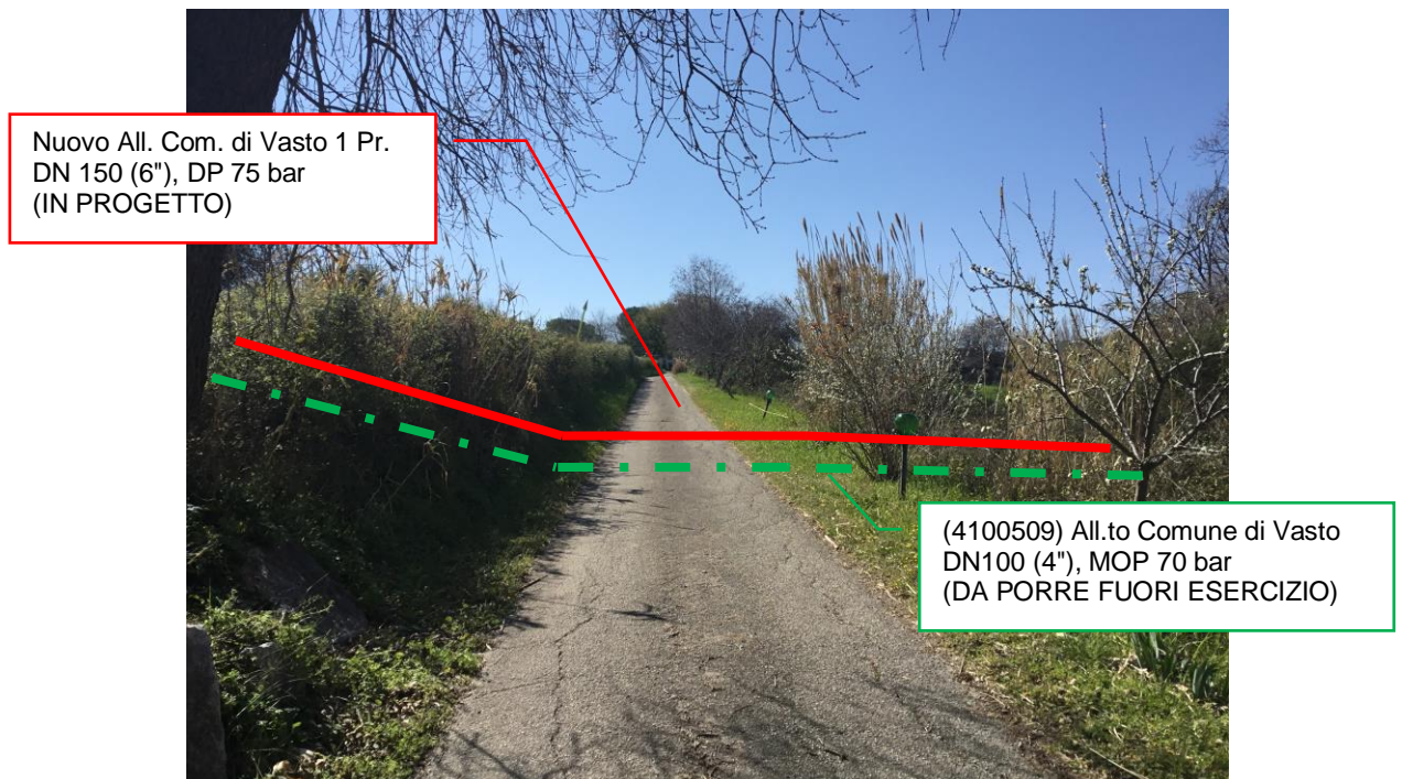
Foto n.4 – Km 0+600 - Metanodotti in progetto e da porre fuori esercizio su strada Via Buonanotte
