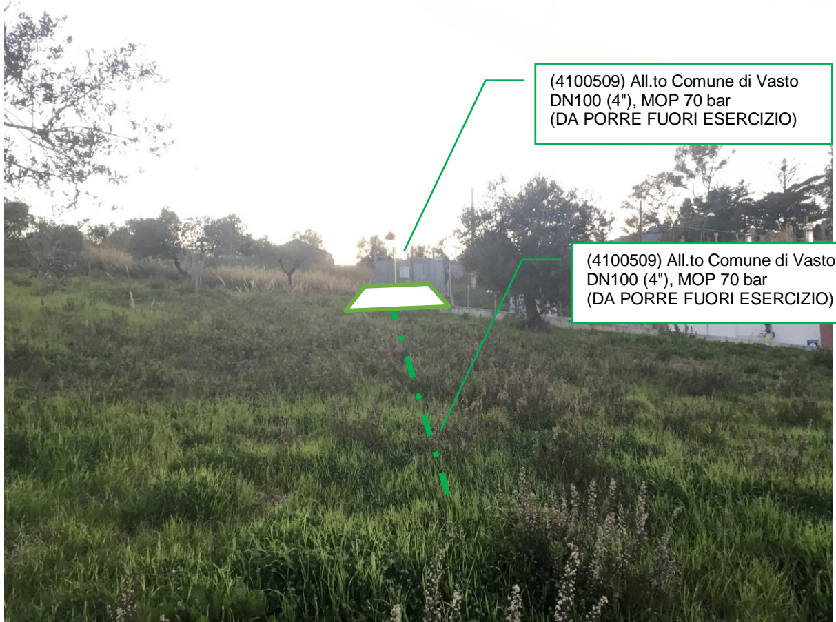
Foto n.11 – km 3+750 - Impianto P.I.D.A. n.2 Com. di Vasto (DA PORRE FUORI ESERCIZIO)
