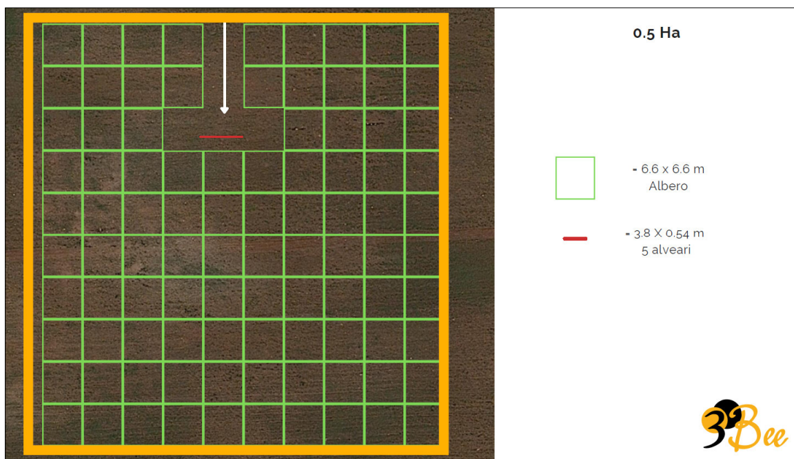
Figura 6 - Schema piantumazione e posizionamento alveari
