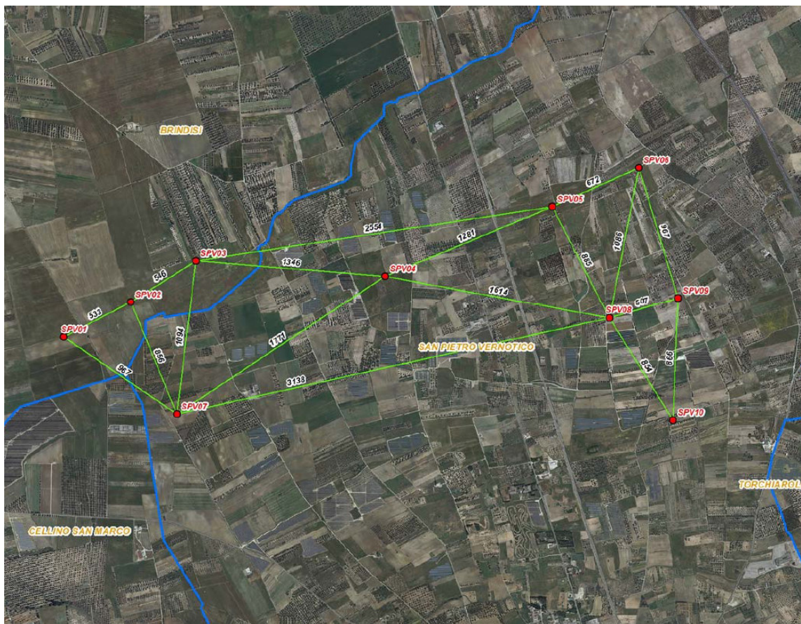
Figura 3 - Distanze tra aerogeneratori
