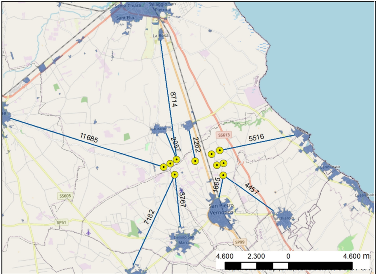
Figura 1 - Distanza aerogeneratori di progetto dai centri abitati limitrofi
