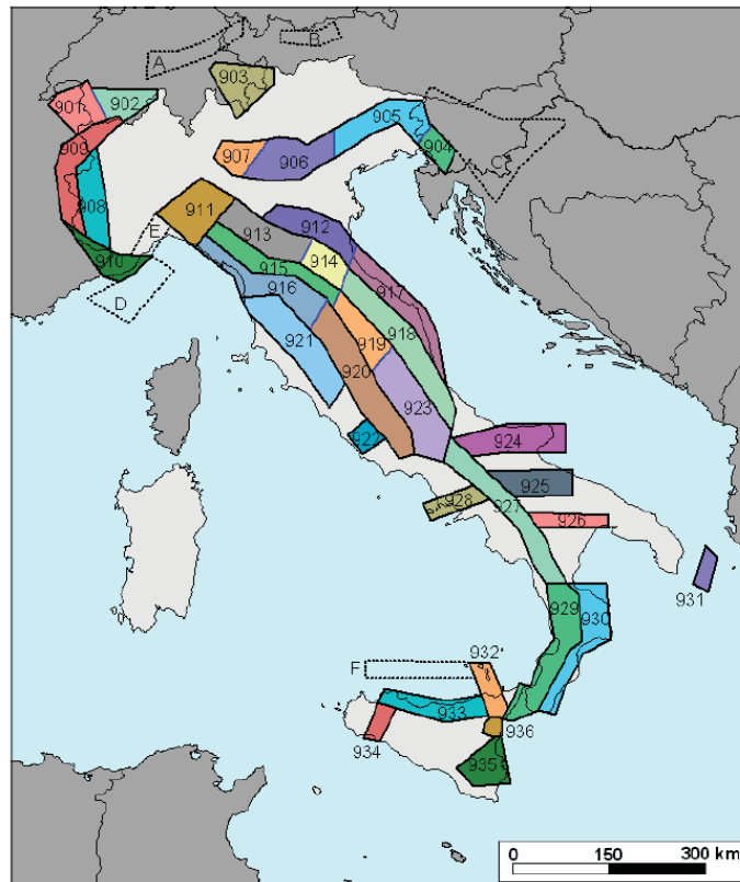
Figura 1 - Zonazione sismogenetica ZS9. Dal sito zonesismiche.mi.ingv.it (Gruppo di Lavoro, 2004)
