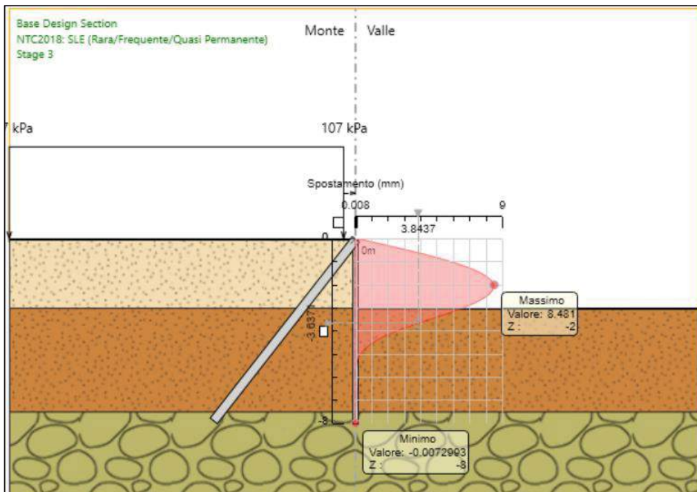
Figura 56 – Spostamenti SLE
