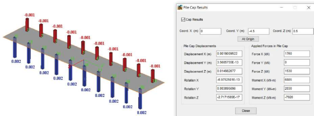
Figura 28 – Cedimenti e rotazioni fondazione
