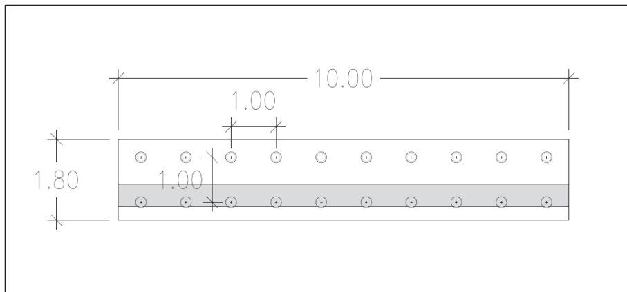
Figura 3: Vista in pianta di un conccio del muro di sottoscarpa di lunghezza 10 m [3]
