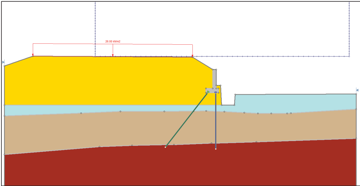
Figura 58 – Sezione 4 – Modello Slide
