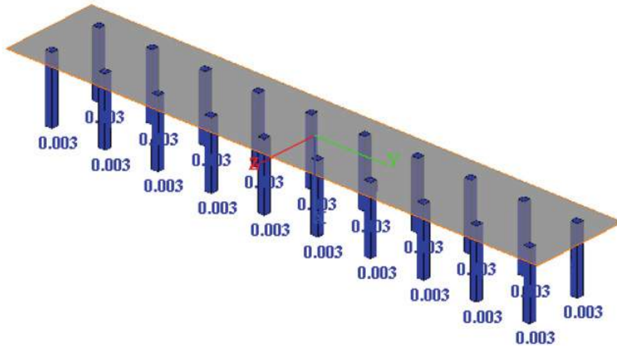
Figura 55 – Spostamenti orizzontali fondazione
