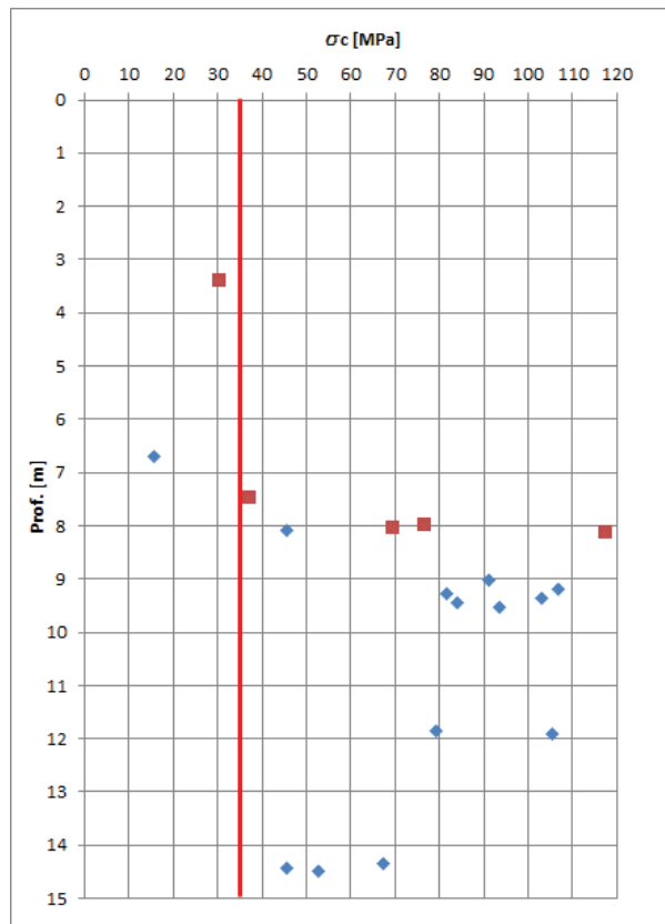
Figura 4 - Unita B – Resistenza a compressione uniassiale
