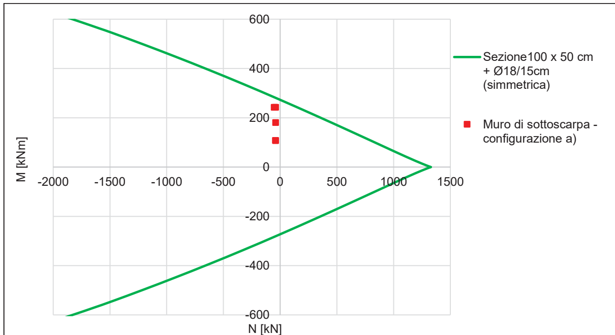
Figura 9: Verifica a pressoflessione dell'elevazione del muro di sottoscarpa – configurazione a)
