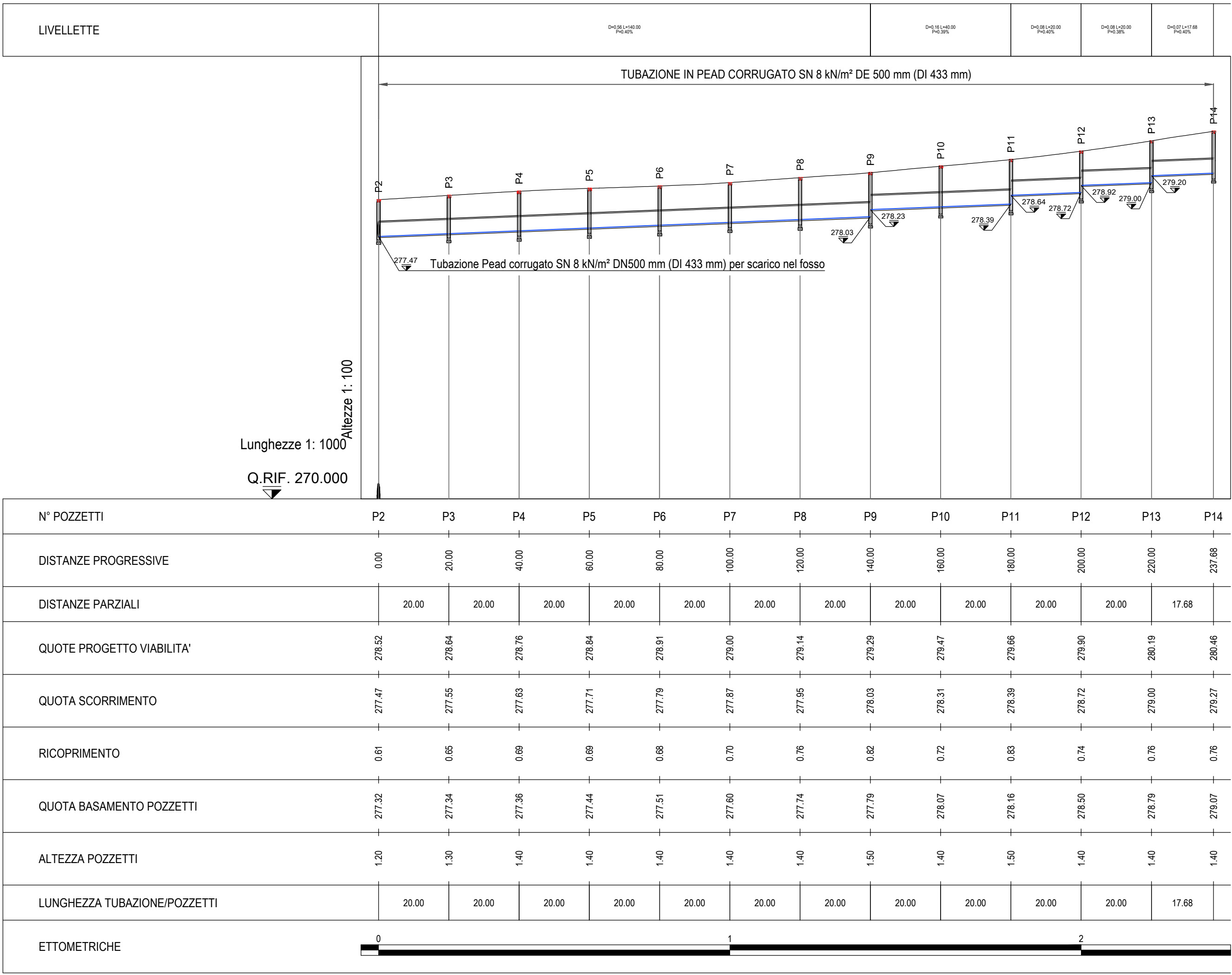
PROFILO LONGITUDINALE SS131 SUD: ASSE POZZETTI P2-P14
