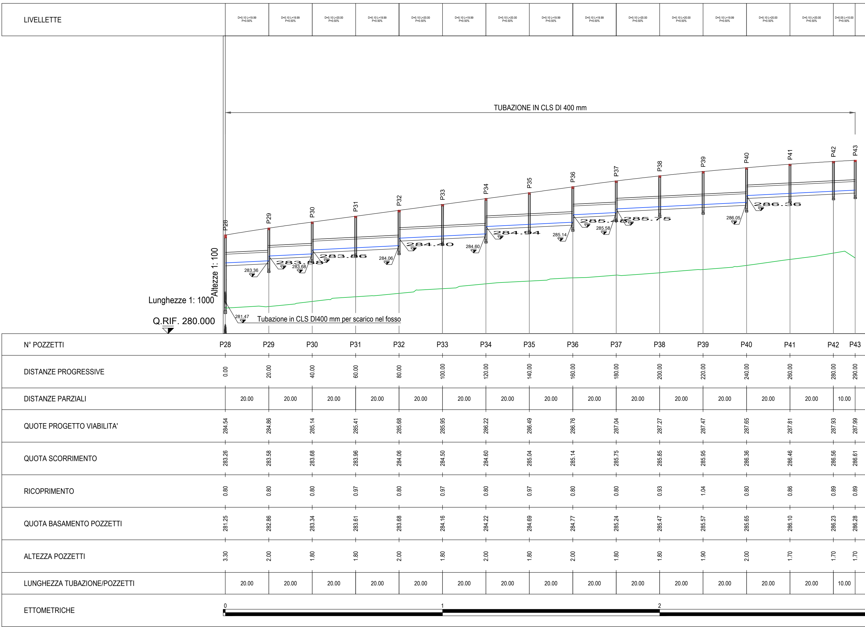
PROFILO LONGITUDINALE SS131 SUD: ASSE POZZETTI P28-P43
