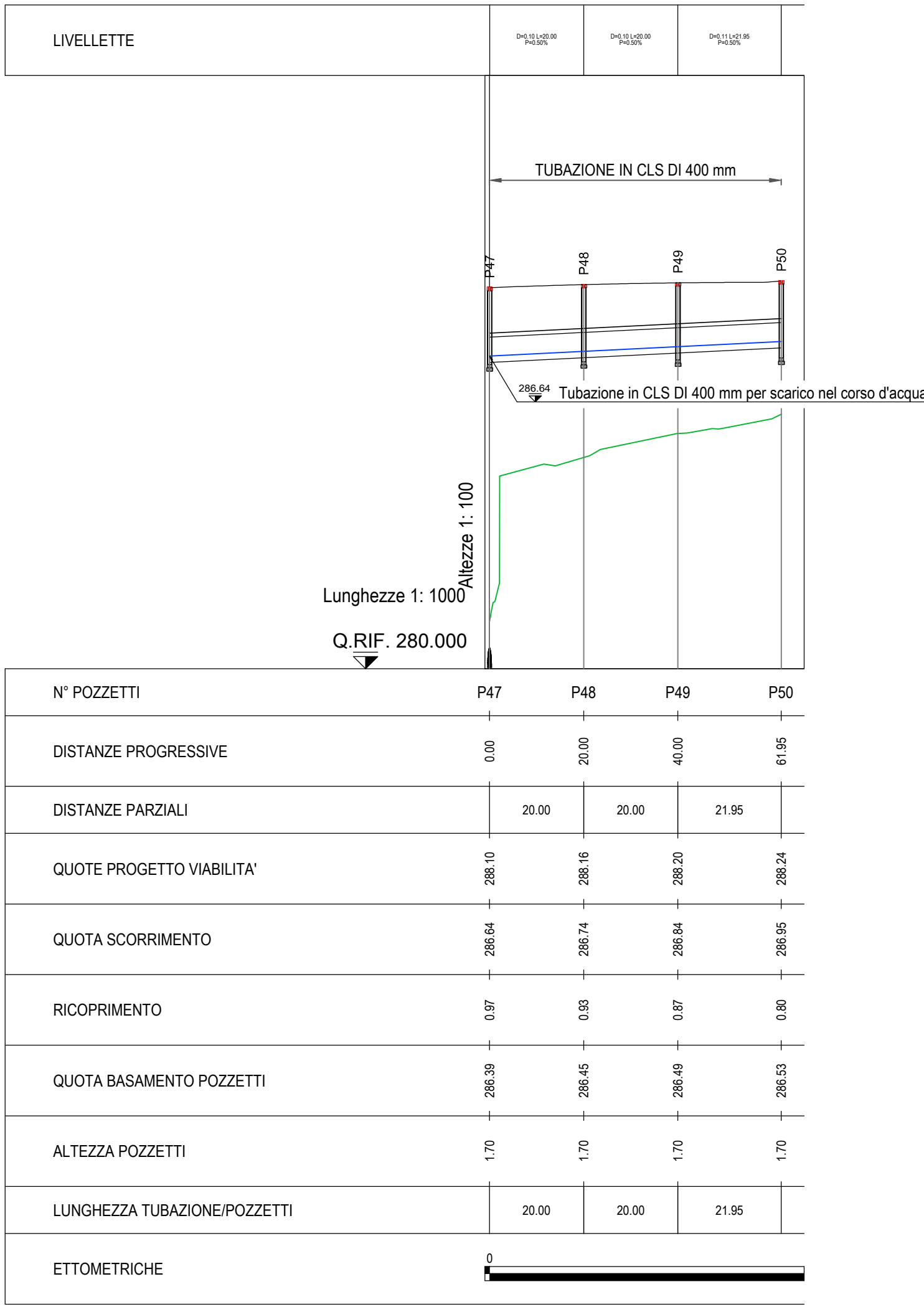
PROFILO LONGITUDINALE SS131 NORD: ASSE POZZETTI P47-P50
