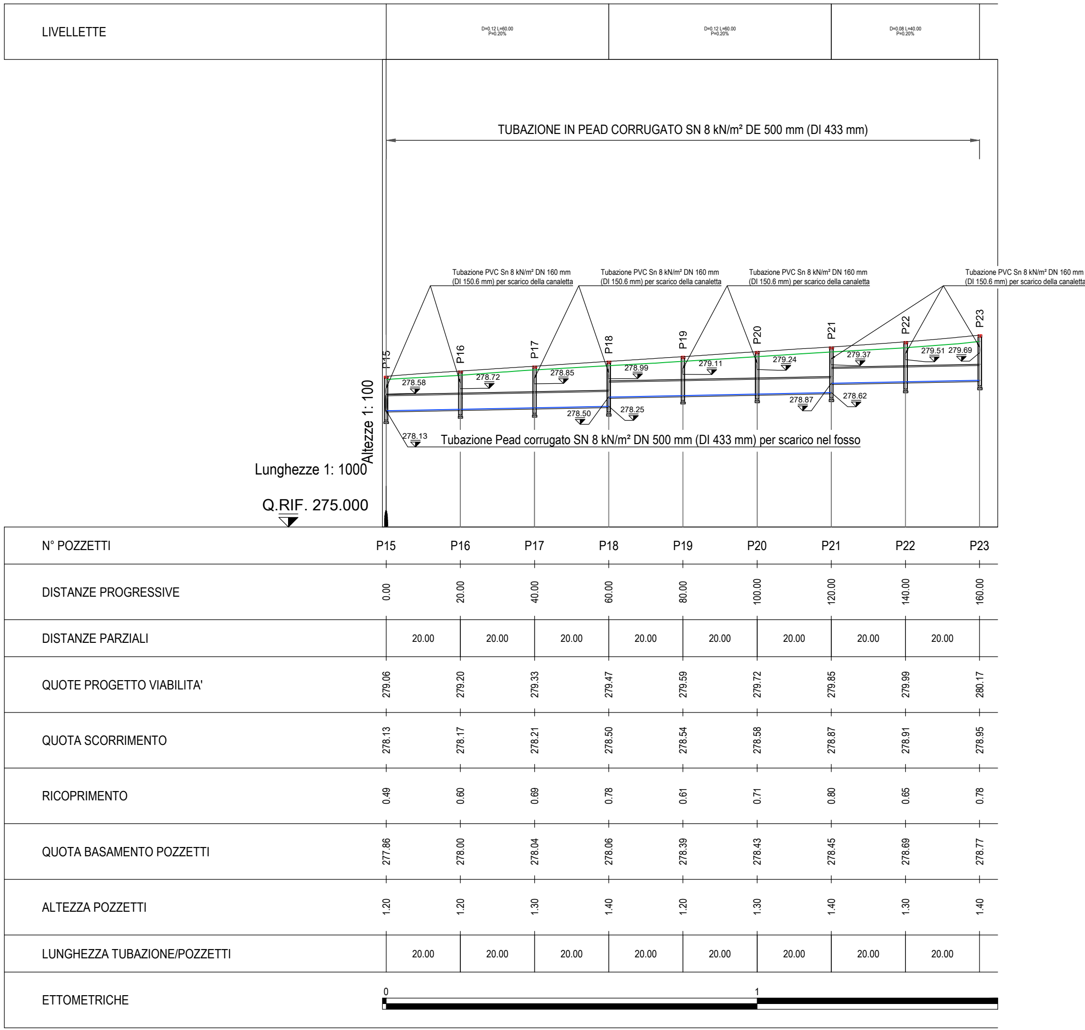
PROFILO LONGITUDINALE SS131 NORD: ASSE POZZETTI P15-P23
