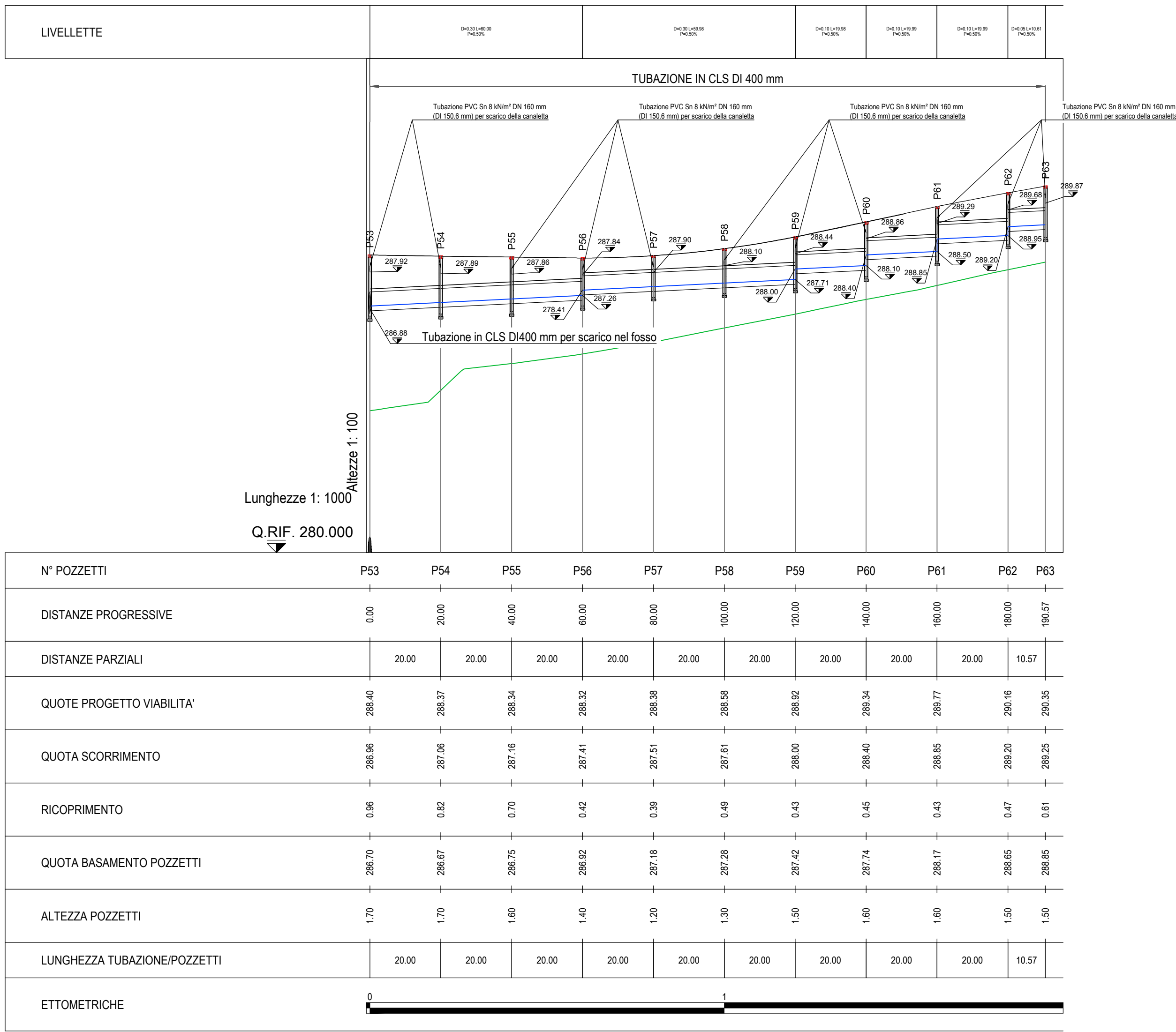
PROFILO LONGITUDINALE SS131 NORD: ASSE POZZETTI P53-P63
