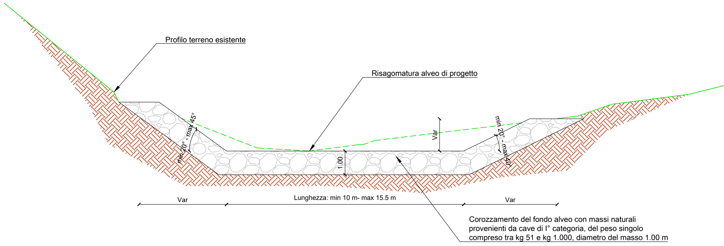
SEZIONE TIPOLOGICA RIPROFILATURA ALVEO scala 1:100
