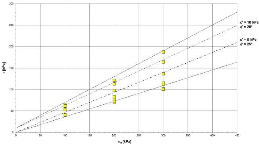
Figura 6 – Involucro di rottura ottenuto da prove di taglio diretto
