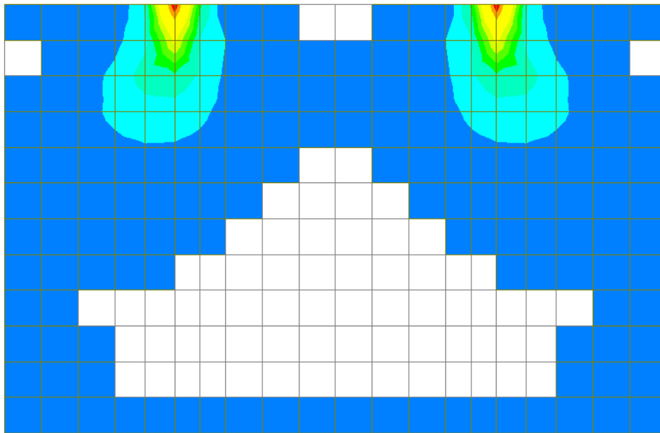
Figura 15-40: Apertura fessure dovuta al momento verticale (-)
