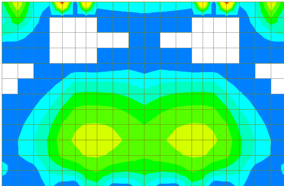
Figura 15-42: Apertura fessure dovuta al momento verticale (+)
