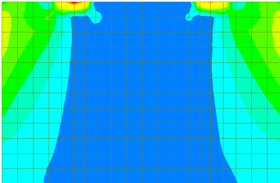
Figura 15-33: Tensioni nel cls dovute al momento flettente orizzontale (-)
