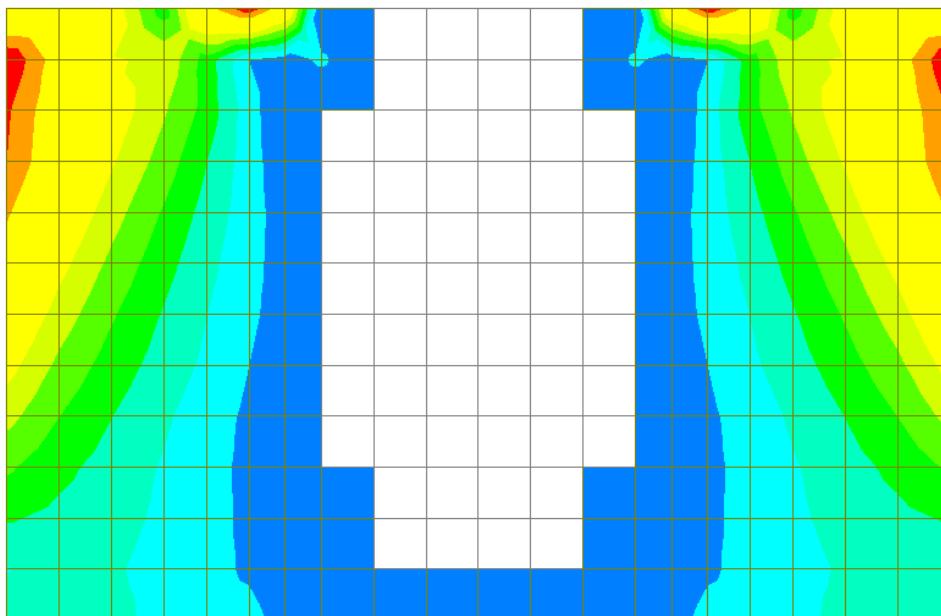
Figura 15-41: Apertura fessure dovuta al momento orizzontale (-)
