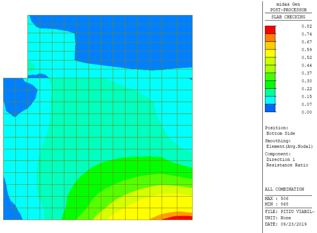
Figura 15-48: Rapporto M_{Sd}/M_{Rd} momento flettente verticale (-): combinazione ENV-SLU
