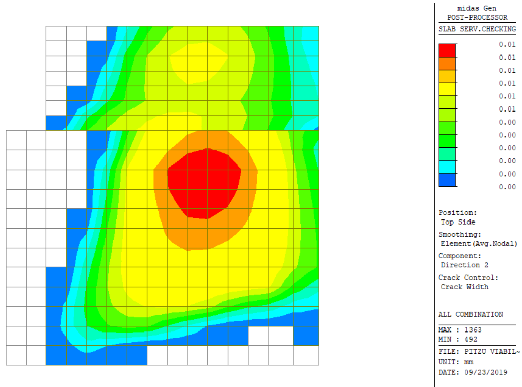
Figura 15-65: Apertura fessure dovuta al momento orizzontale (+)
