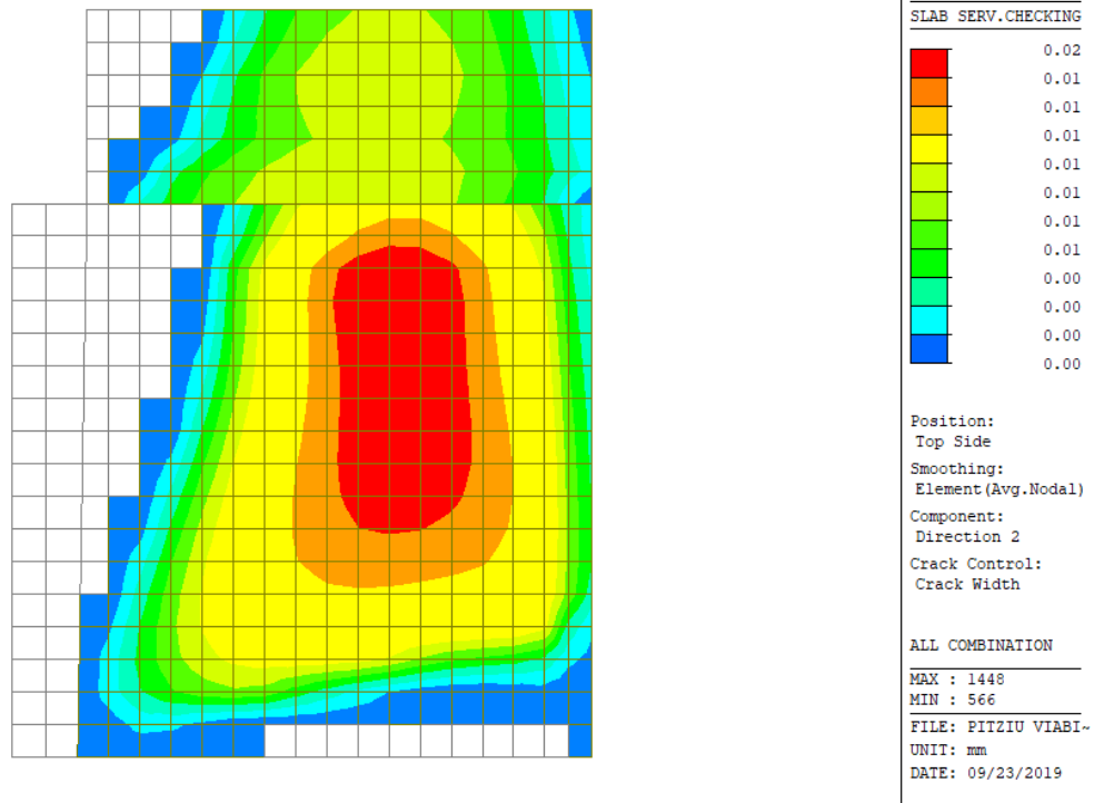
Figura 15-65: Apertura fessure dovuta al momento orizzontale (+)
