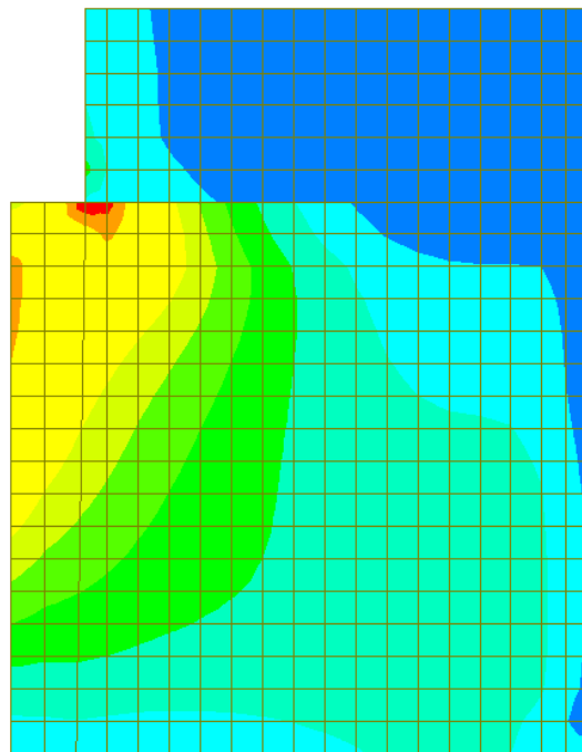
Figura 15-45: Momento flettente orizzontale (-): combinazione ENV-SLU
