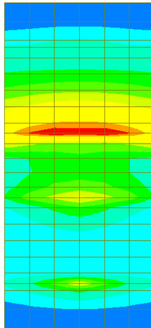
Figura 13-8: Tensioni nel cls dovute al momento flettente My (-)
