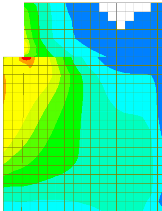
Figura 15-63: Apertura fessure dovuta al momento orizzontale (-)
