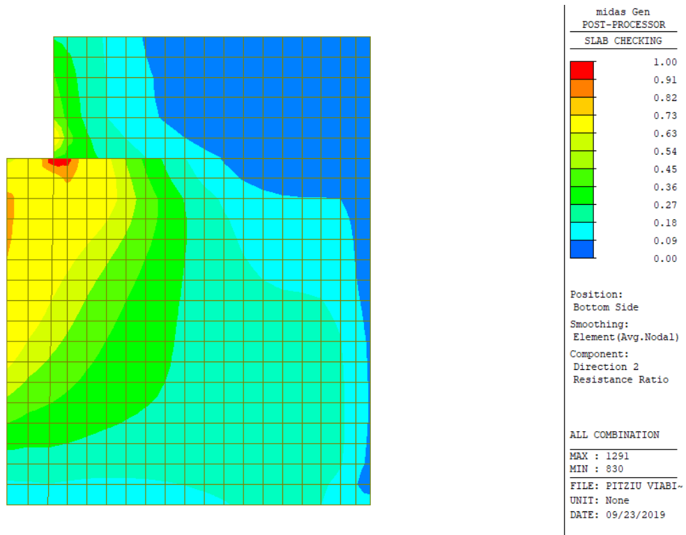
Figura 15-49: Rapporto M_{Sd}/M_{Rd} momento flettente orizzontale (-): combinazione ENV-SLU
