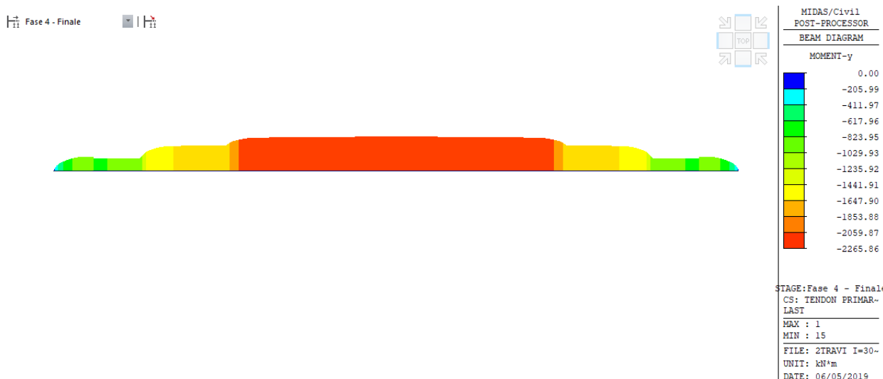
Figura 12-6 Effetto della precompressione – Sollecitazioni di momento flettente
