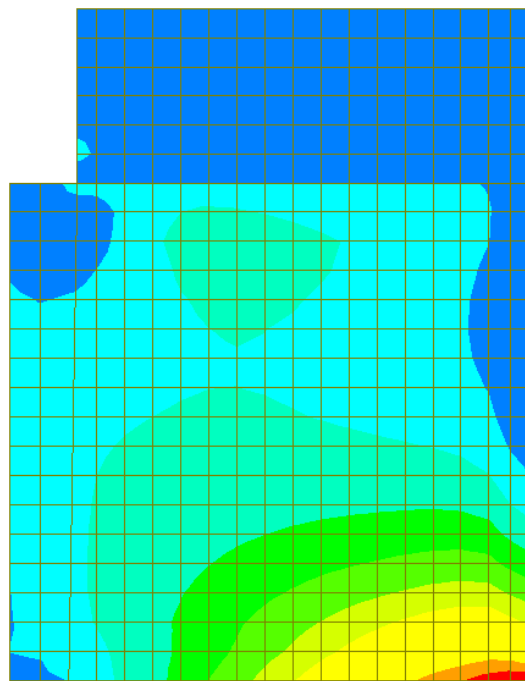
Figura 15-44: Momento flettente verticale (-): combinazione ENV-SLU
