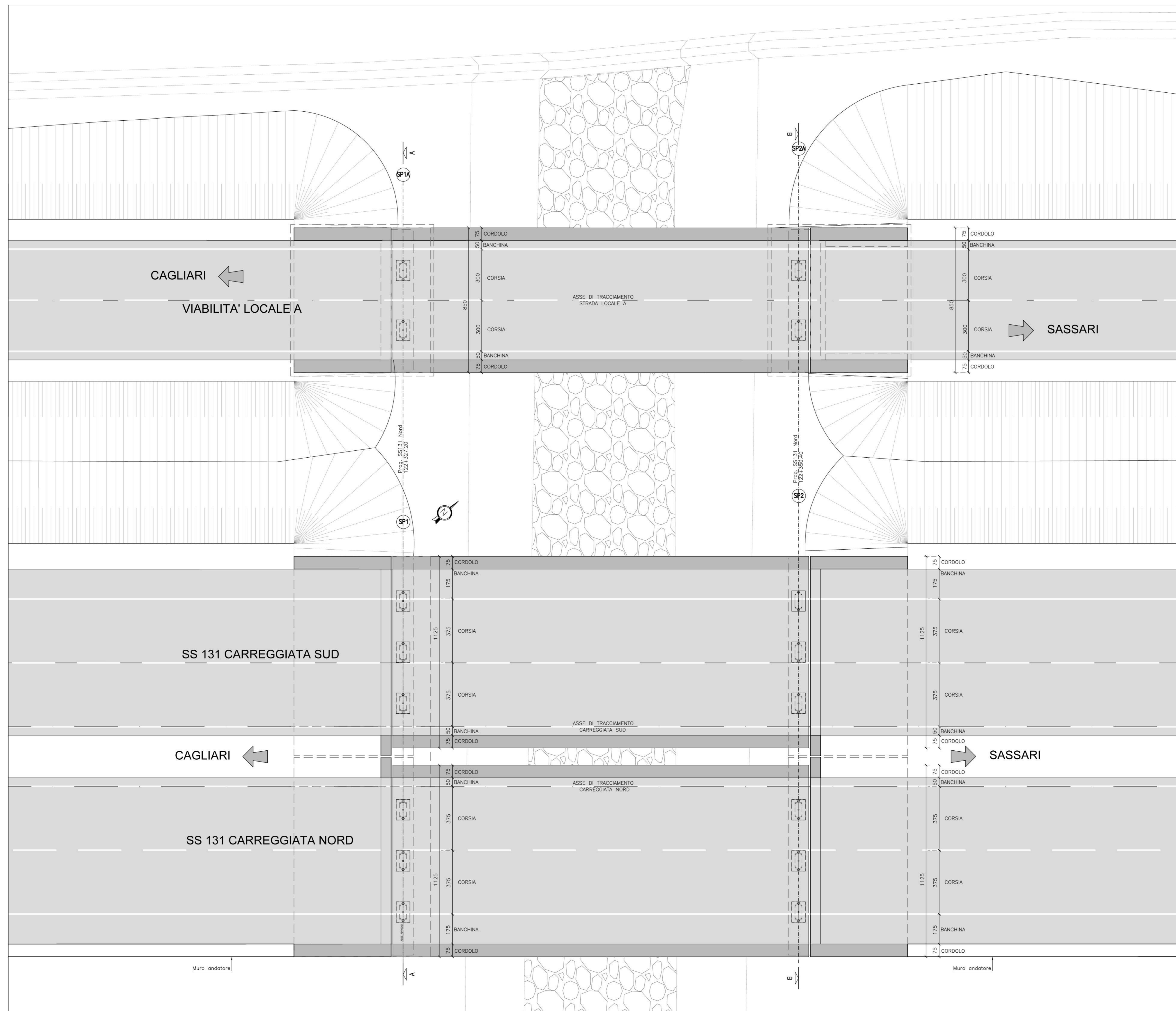
PIANTA Scala 1:100
