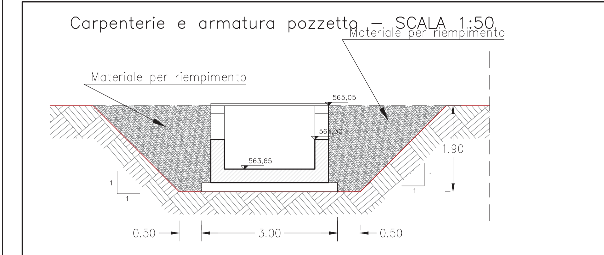
Sezione trasversale pozzetto imbocco Tombino TC12 – SCALA 1:50
