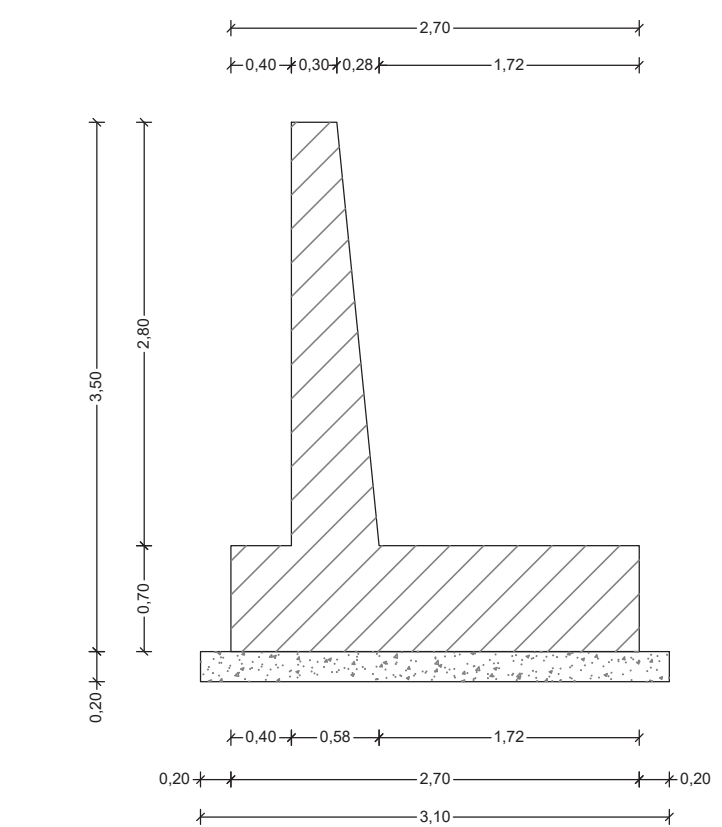
SEZIONE C - C SCALA 1:50
