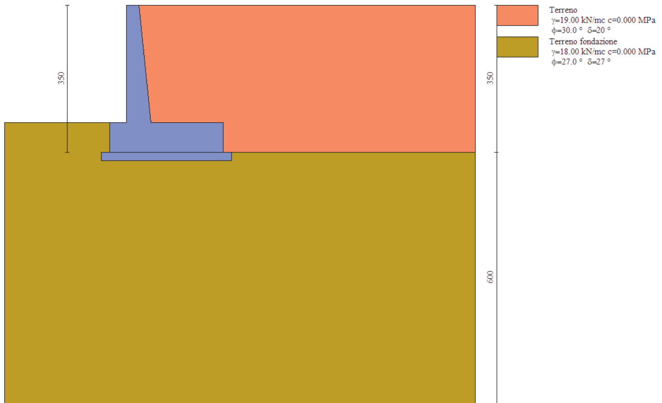
Figura 21 – Profilo del terreno
