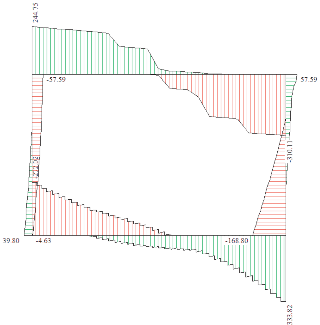
Figura 16 – Inviluppo del diagramma del taglio
