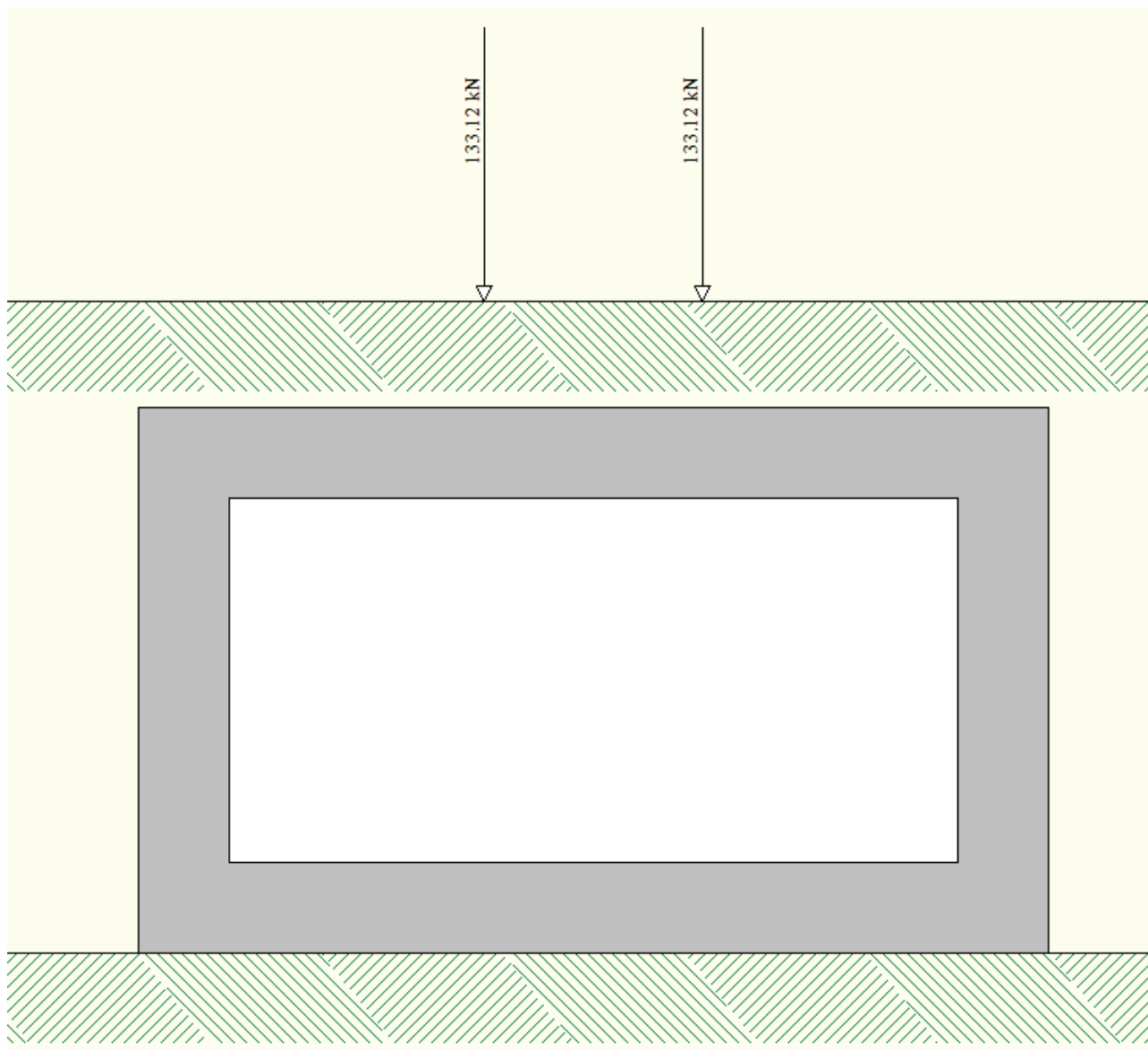
Figura 9 – Gruppo 1 – carico tandem (condizione di carico n°8)
