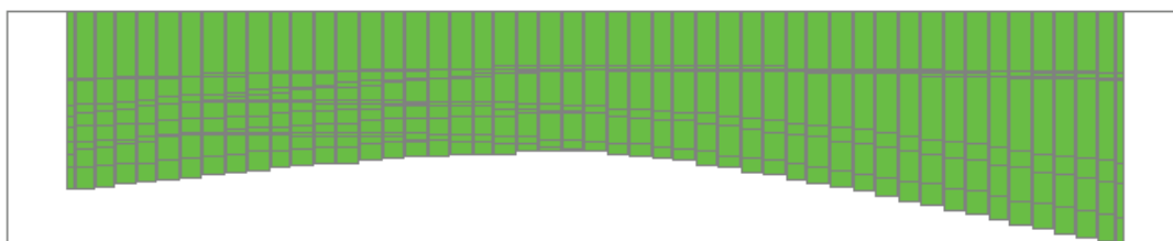
Figura 18 – Involuppo delle pressioni sul terreno di fondazione
