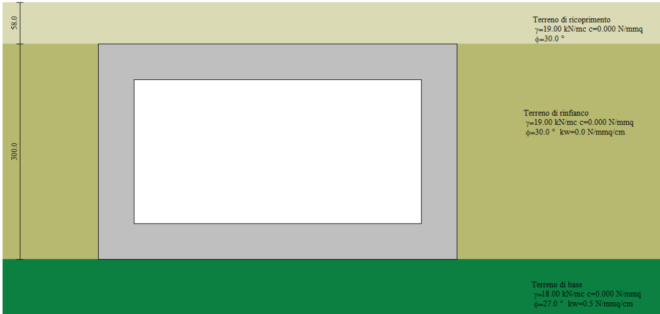
Figura 2 – Stratigrafia e caratteristiche del terreno
