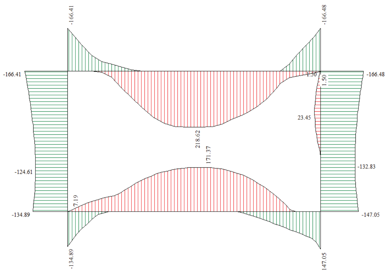
Figura 15 – Inviluppo del diagramma del momento
