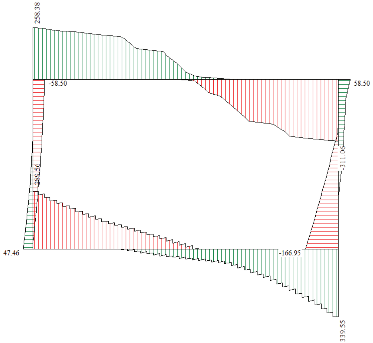
Figura 16 – Inviluppo del diagramma del taglio
