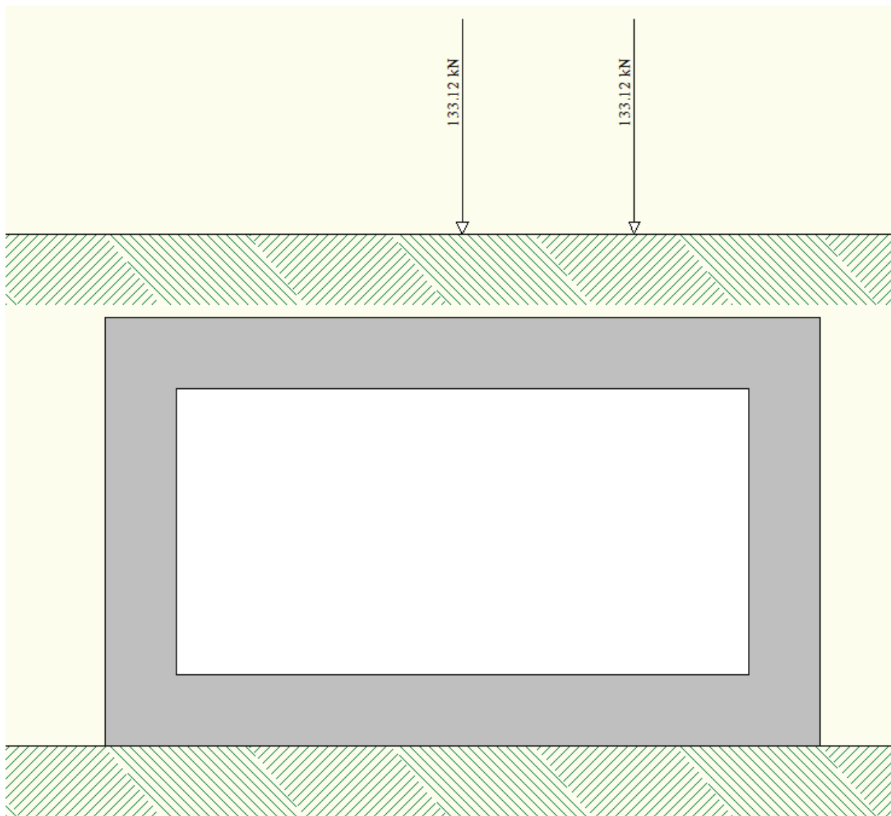
Figura 11 – Gruppo 2 – carico tandem (condizione di carico n°9)
