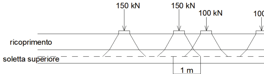
Figura 7 – Diffusione trasversale dei carichi tandem
