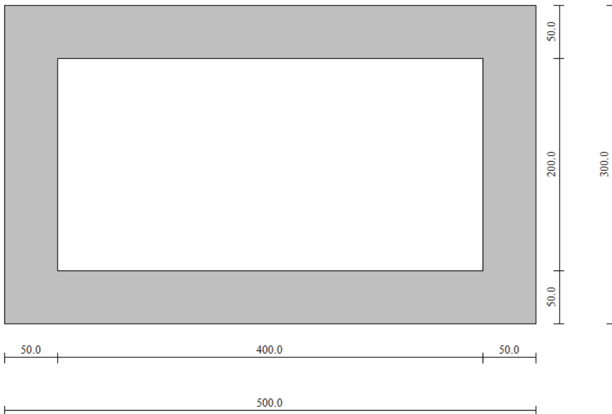
Figura 1 – Sezione trasversale del tombino
