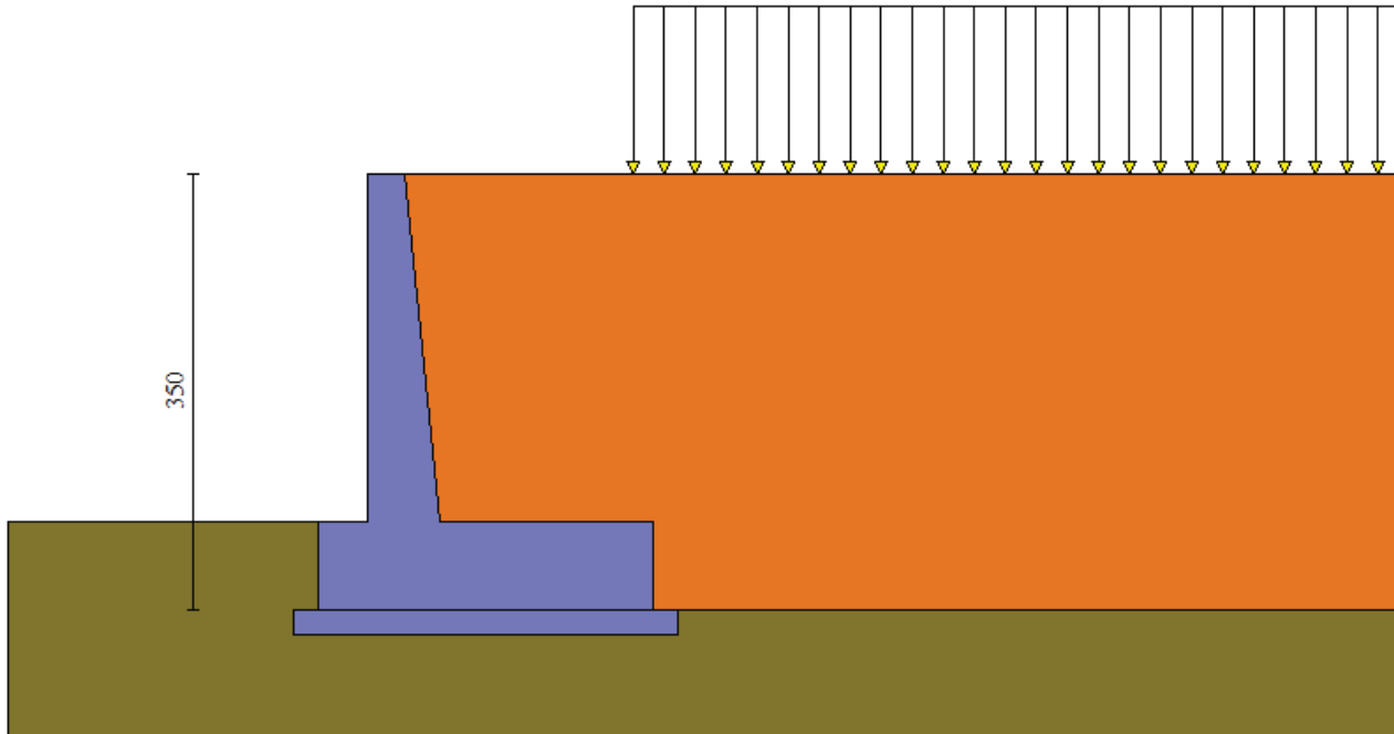
Figura 22 – Carico variabile
