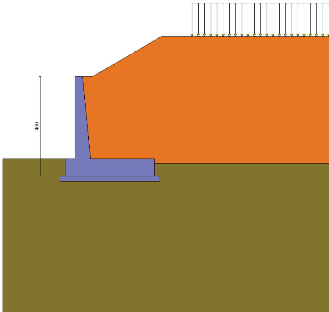
Figura 21 – Carico variabile
