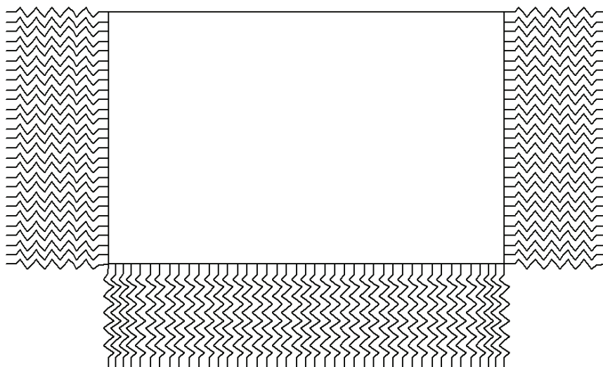
Figura 3 – Schematizzazione del terreno mediante molle
