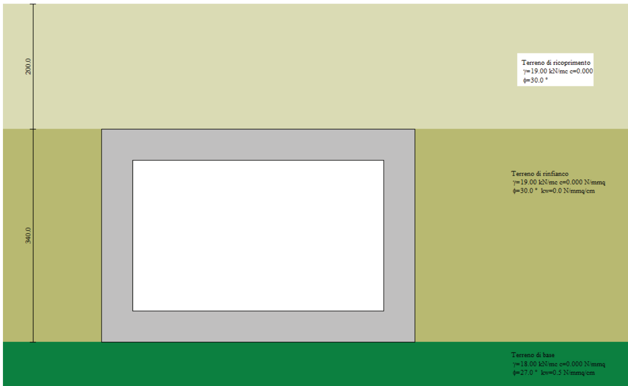
Figura 2 – Stratigrafia e caratteristiche del terreno
