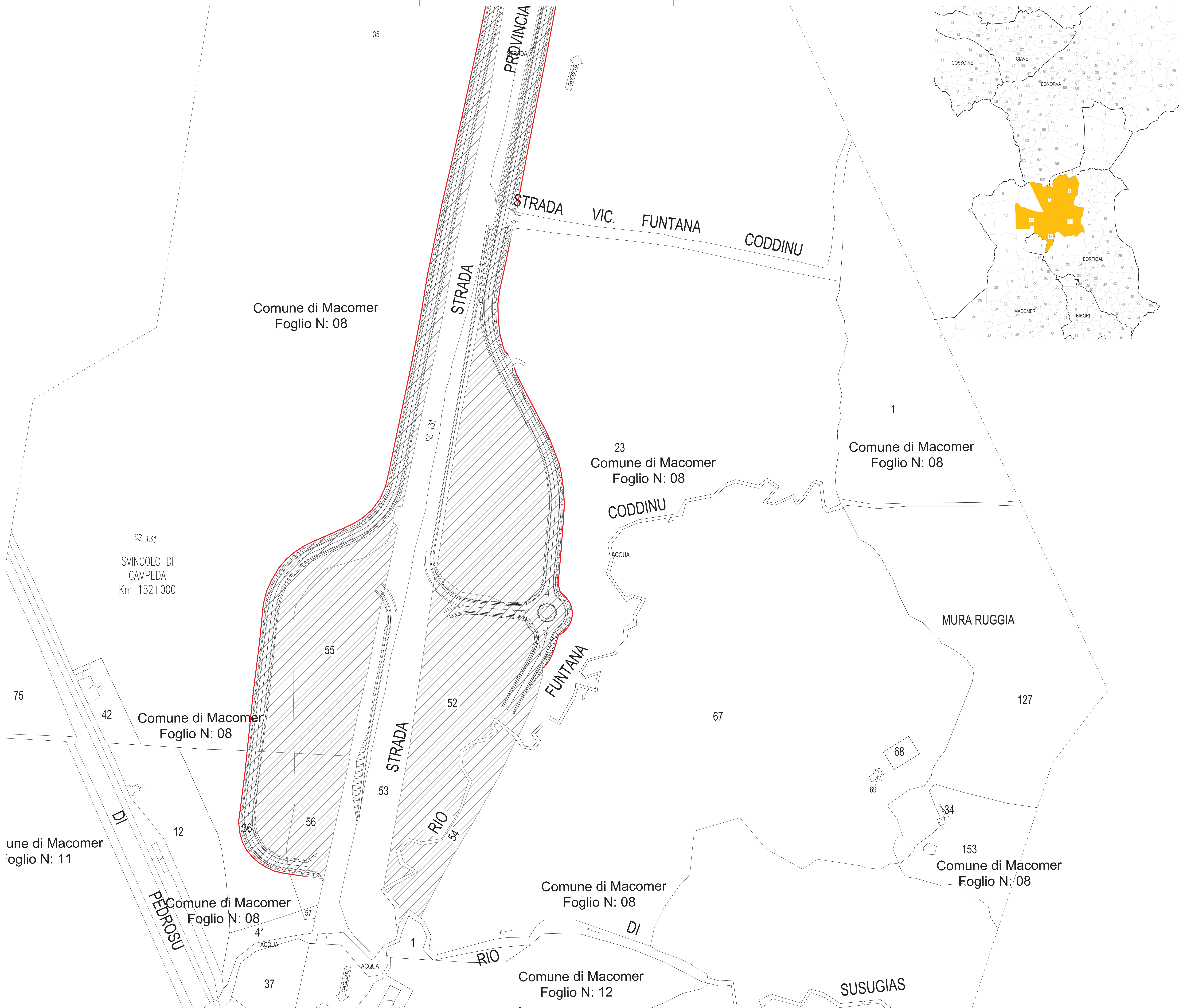
KEY-PLAN
