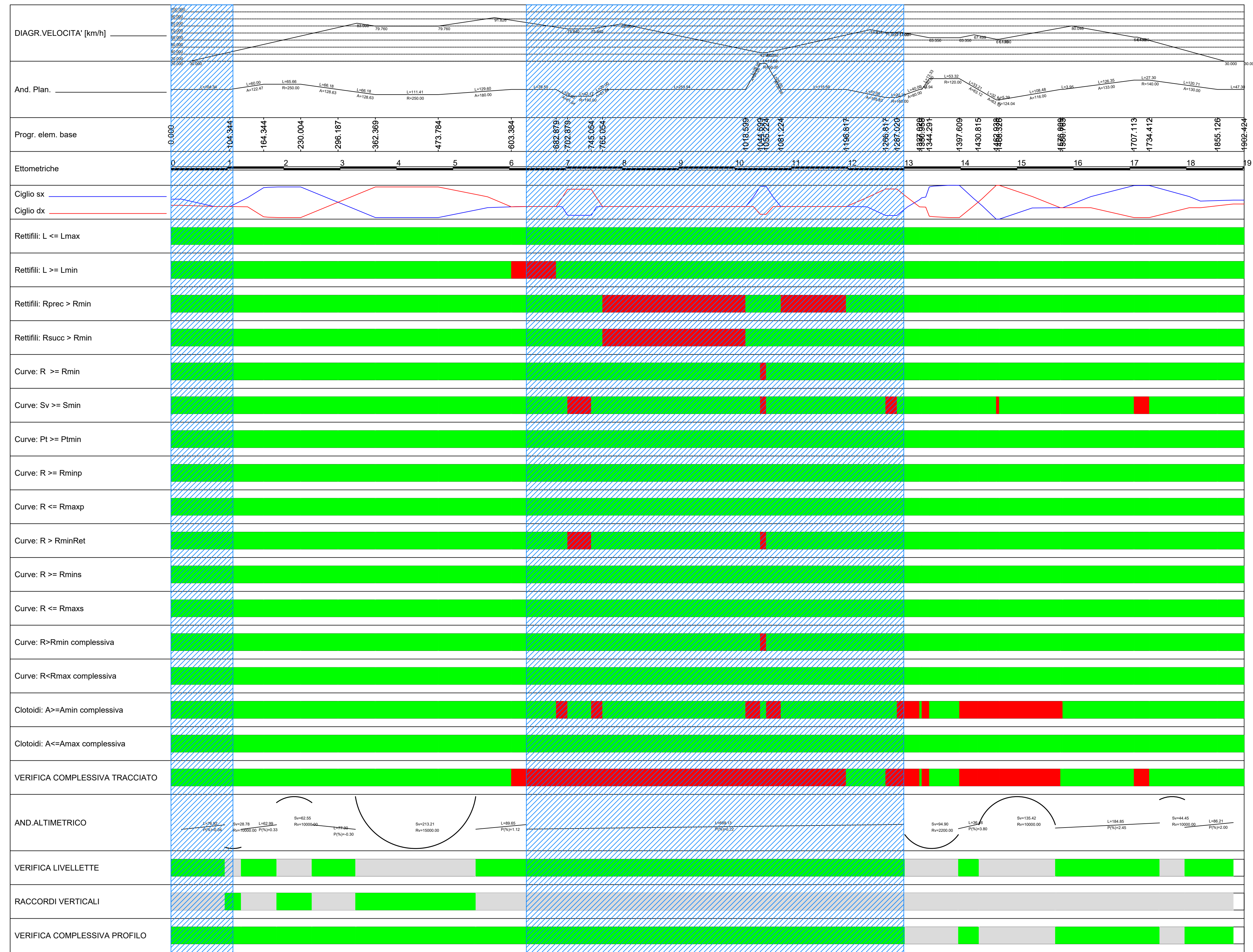
DIAGRAMMA DI VELOCITA' (FLUSSO LIBERO) E VERIFICHE Scala 1: 2000.000
