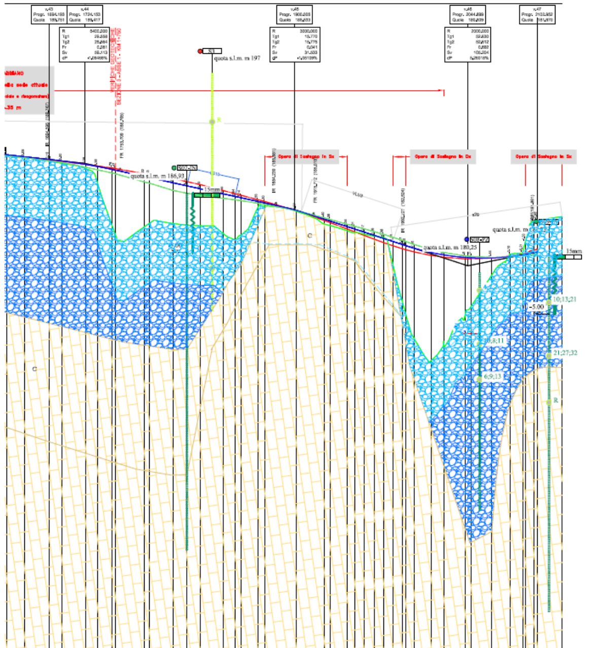
Figura 4: stralcio del profilo geotecnico dell'asse 1
