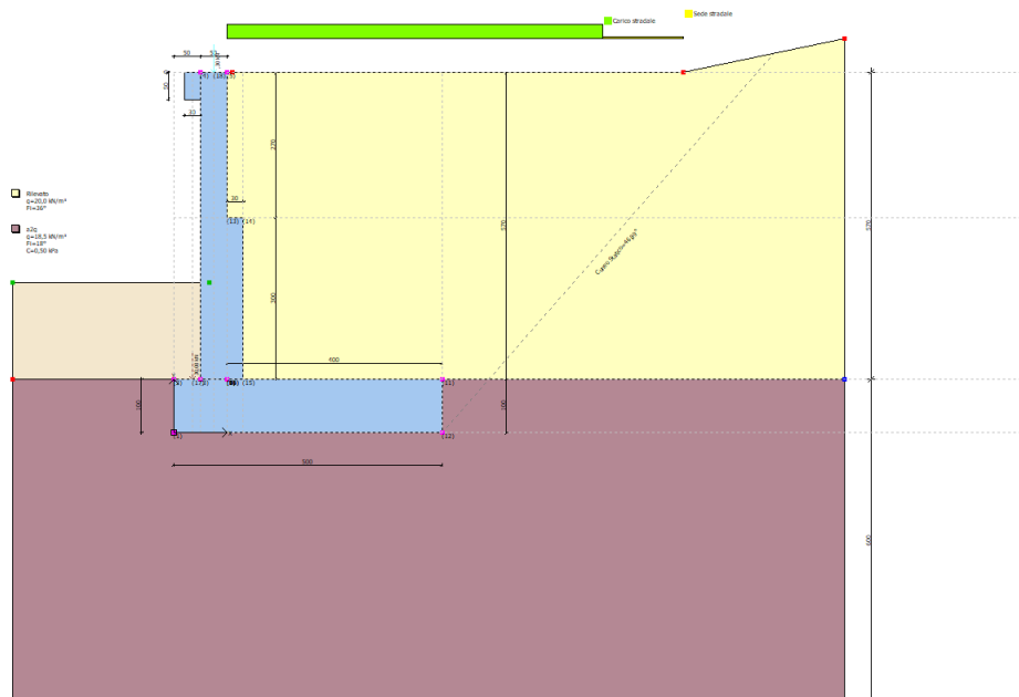
Fig. 7a Modello di calcolo concio 3
