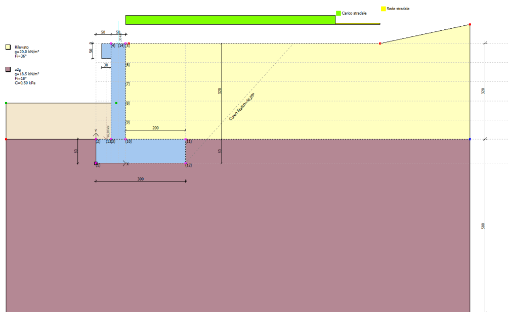
Fig. 7b Modello di calcolo concio 6
