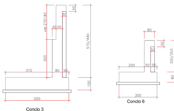
Fig. 1 Sezioni trasversali: concio 3 e concio 6
