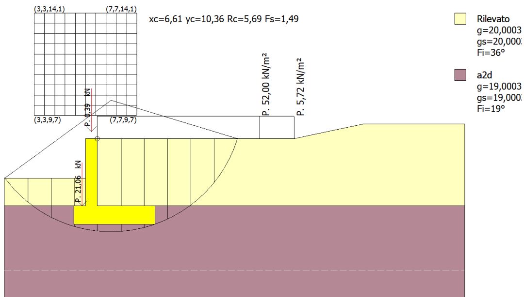
Fig. 9a Modello di calcolo concio 7 (condizione statica)
