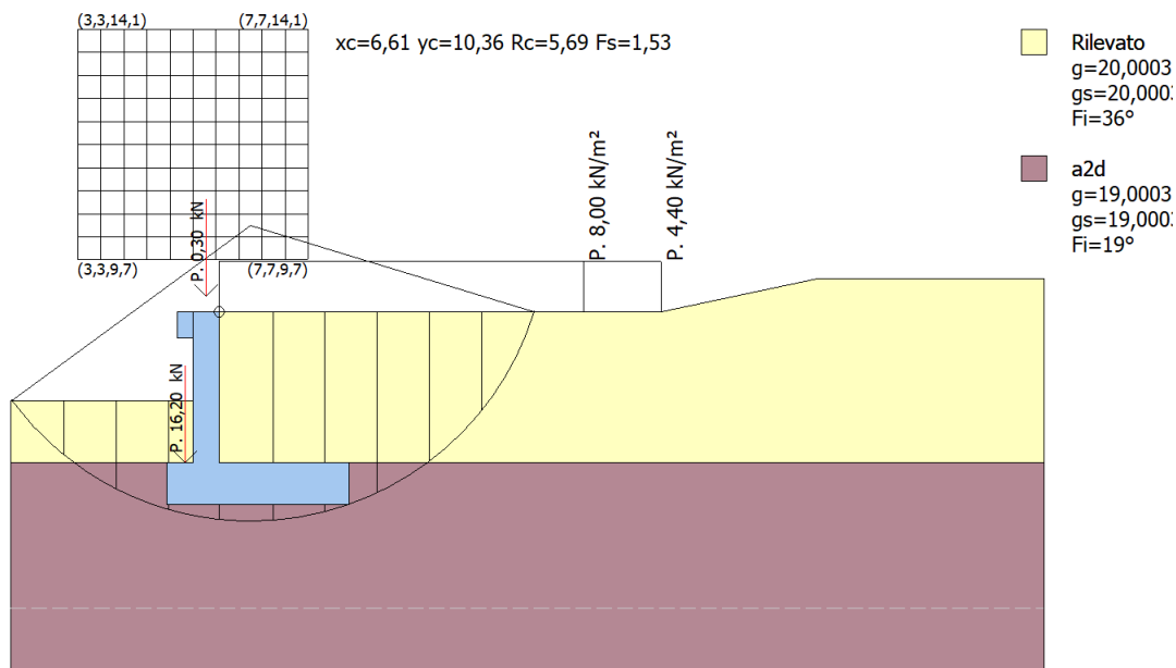
Fig. 9a Modello di calcolo concio 7 (condizione sismica)
