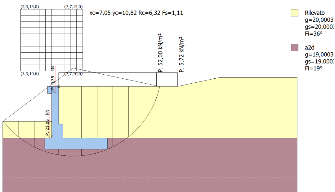
Fig. 8a Modello di calcolo concio 1 (condizione statica)
