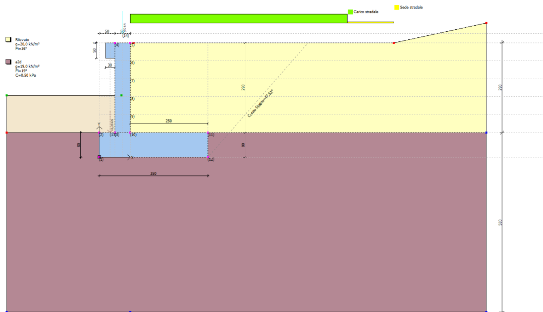
Fig. 7b Modello di calcolo concio 7
