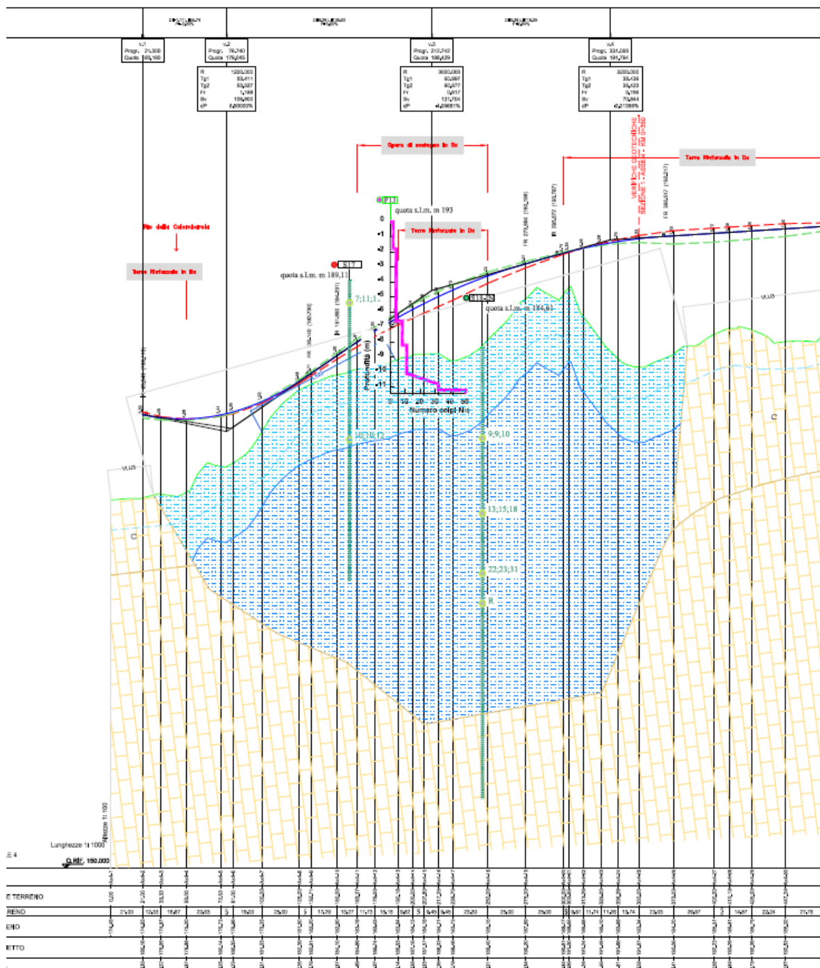
Figura 4: stralcio del profilo geotecnico dell'asse 4
