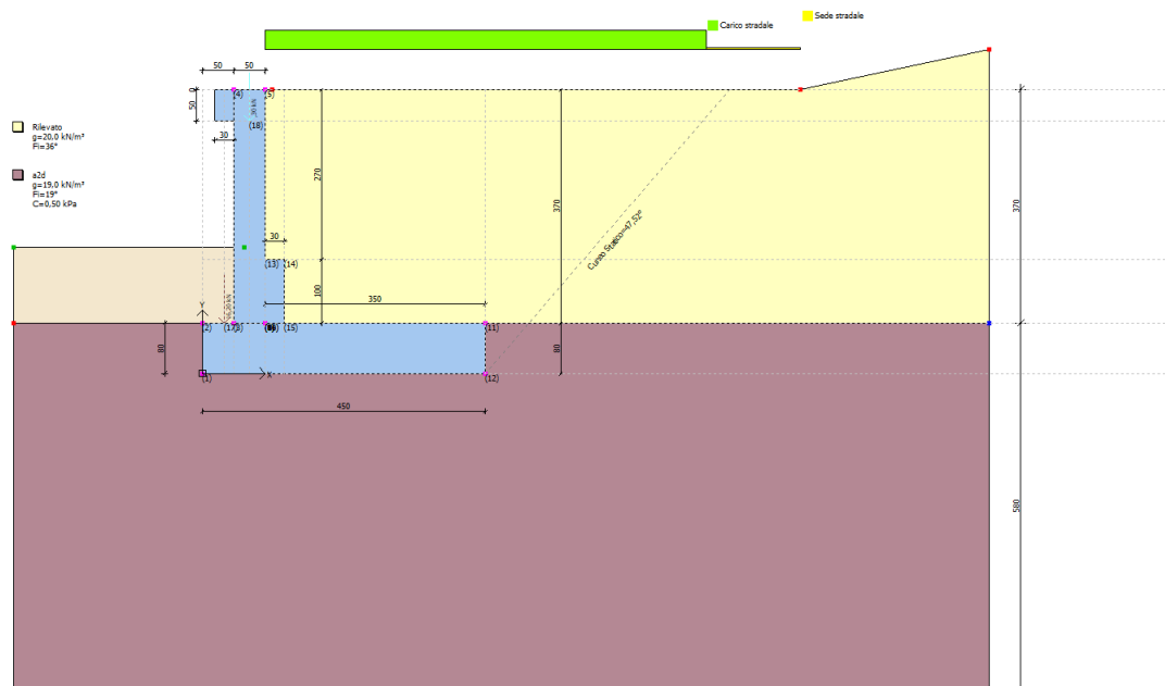
Fig. 7a Modello di calcolo concio 1
