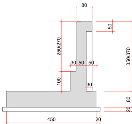
Fig. 1 Sezioni trasversali: concio 1 e concio 7
