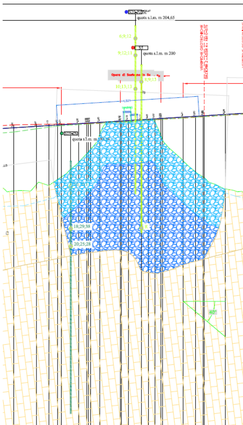
Figura 4: stralcio del profilo geotecnico dell'asse 4
