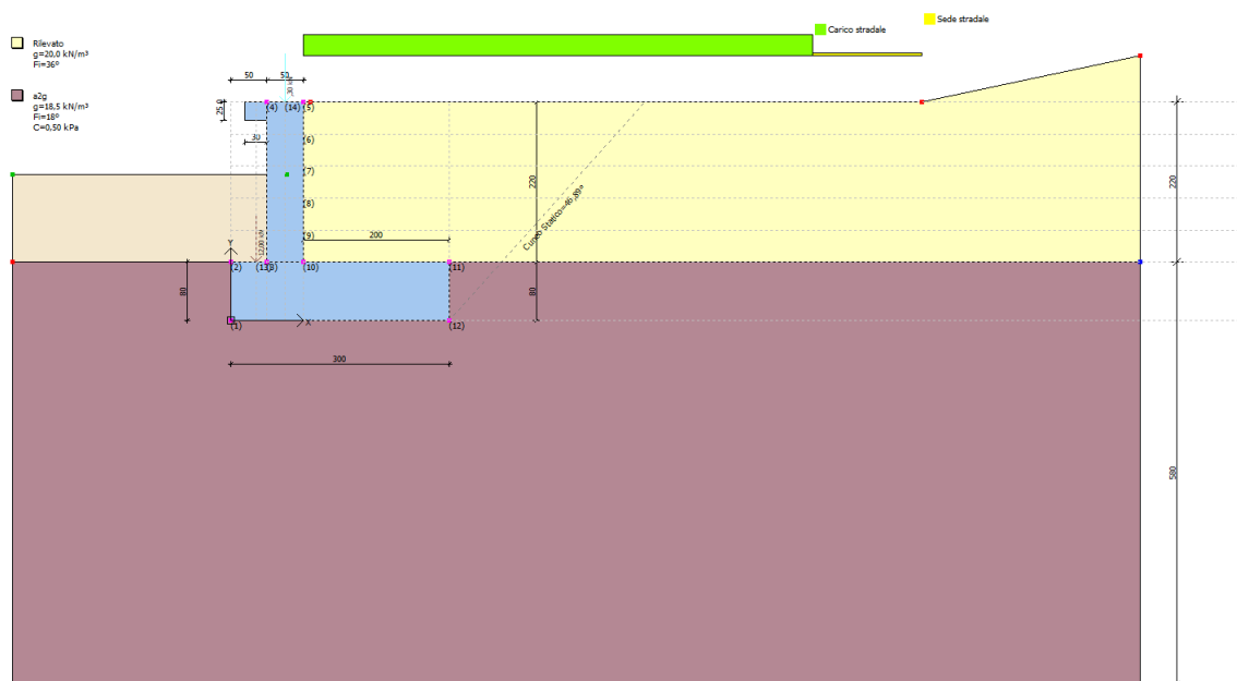
Fig. 7a Modello di calcolo concio tipo
