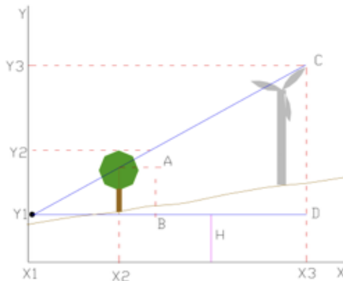
Figura 2-31: Schermatura di una turbina eolica
