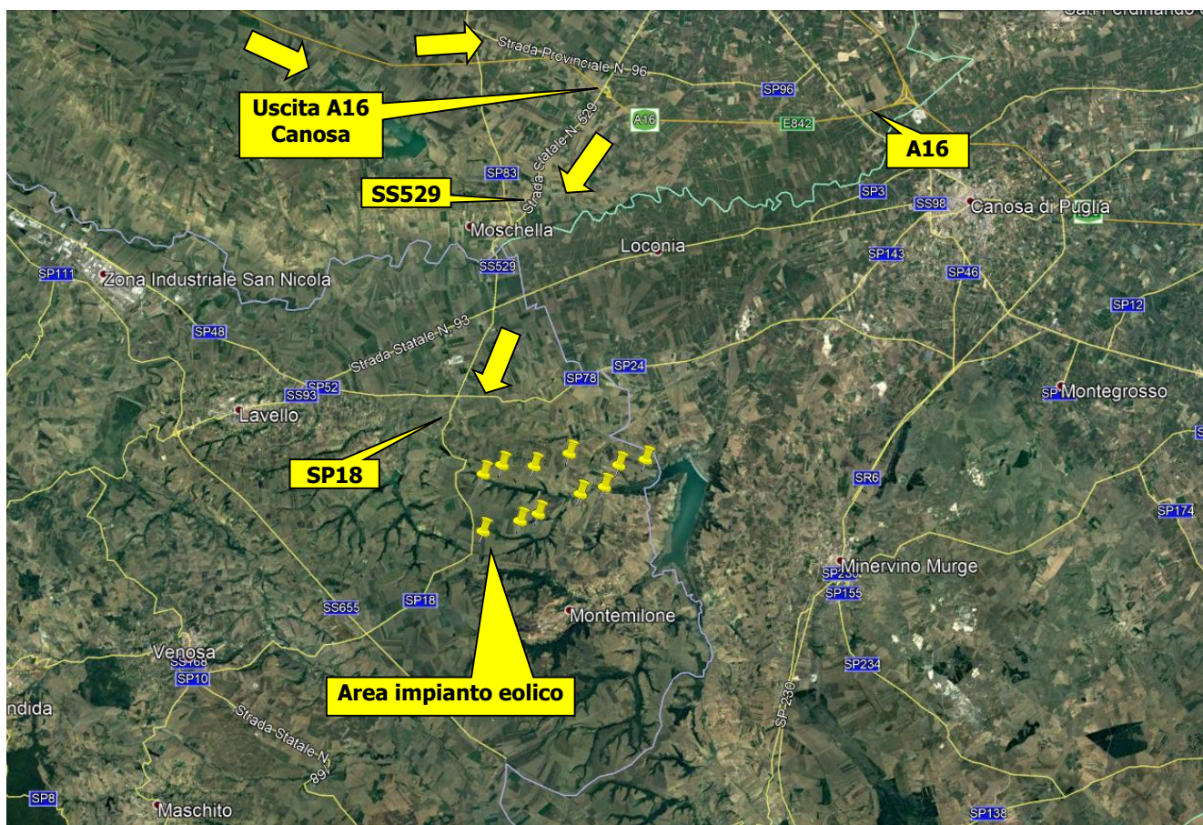
Figura 2-2: Viabilità principale di accesso al sito
