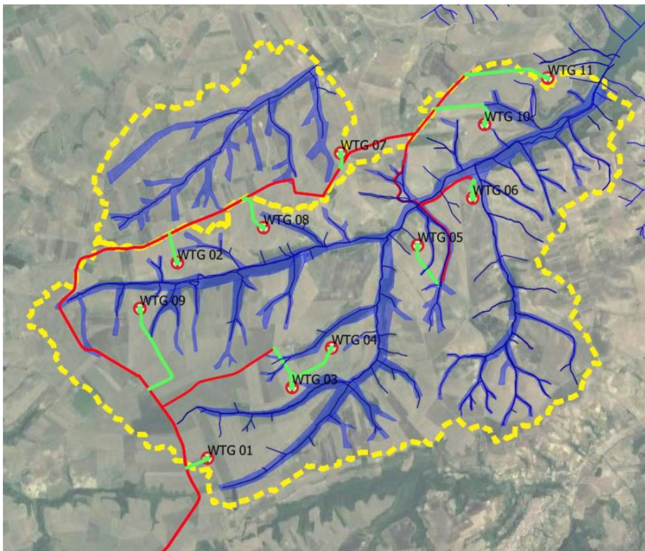
Figura 2-12: Inquadramento rispetto alle aree a pericolosità determinate dallo studio idraulico (ai sensi del PAI Puglia)
