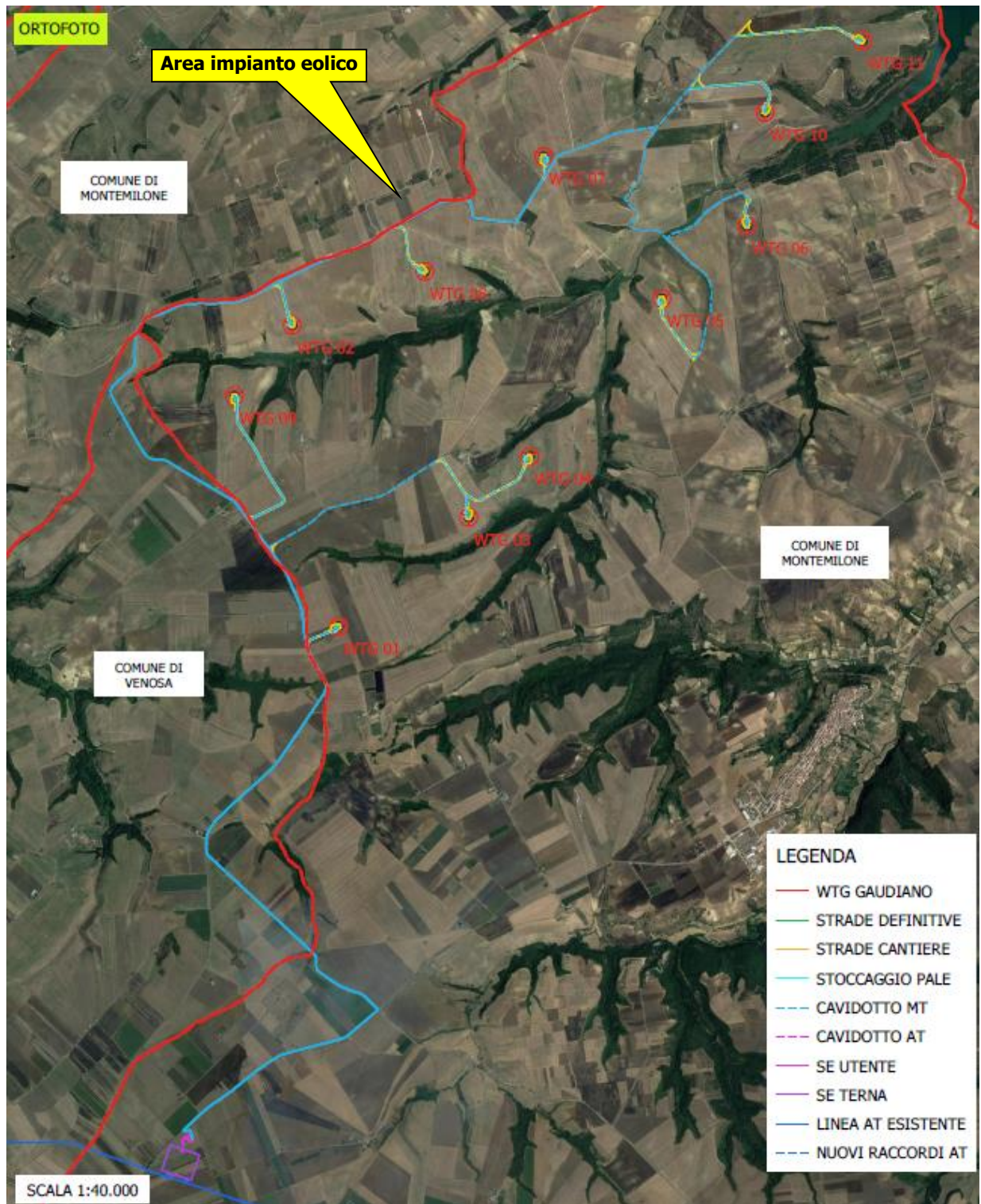
Figura 2-1: Inquadramento intervento di area vasta su ortofoto
