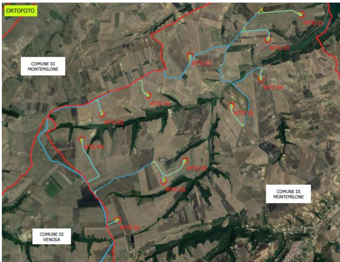
Figura 2-24: inquadramento dell'impianto eolico
