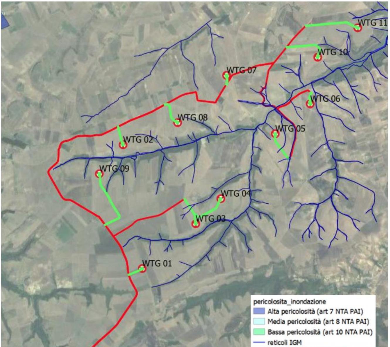
Figura 2-10: Inquadramento intervento su ortofoto rispetto le aree a diversa pericolosità idraulica riportate nel PAI vigente
