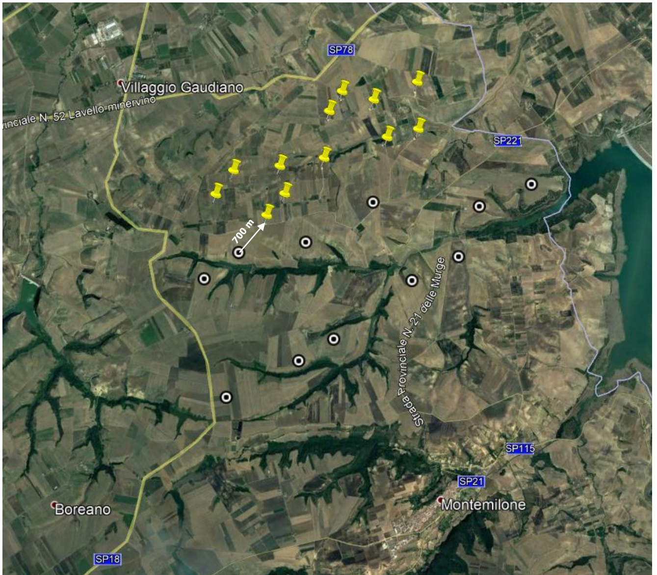
Figura 4-7: Distanza minima tra le turbine delle iniziative presenti
