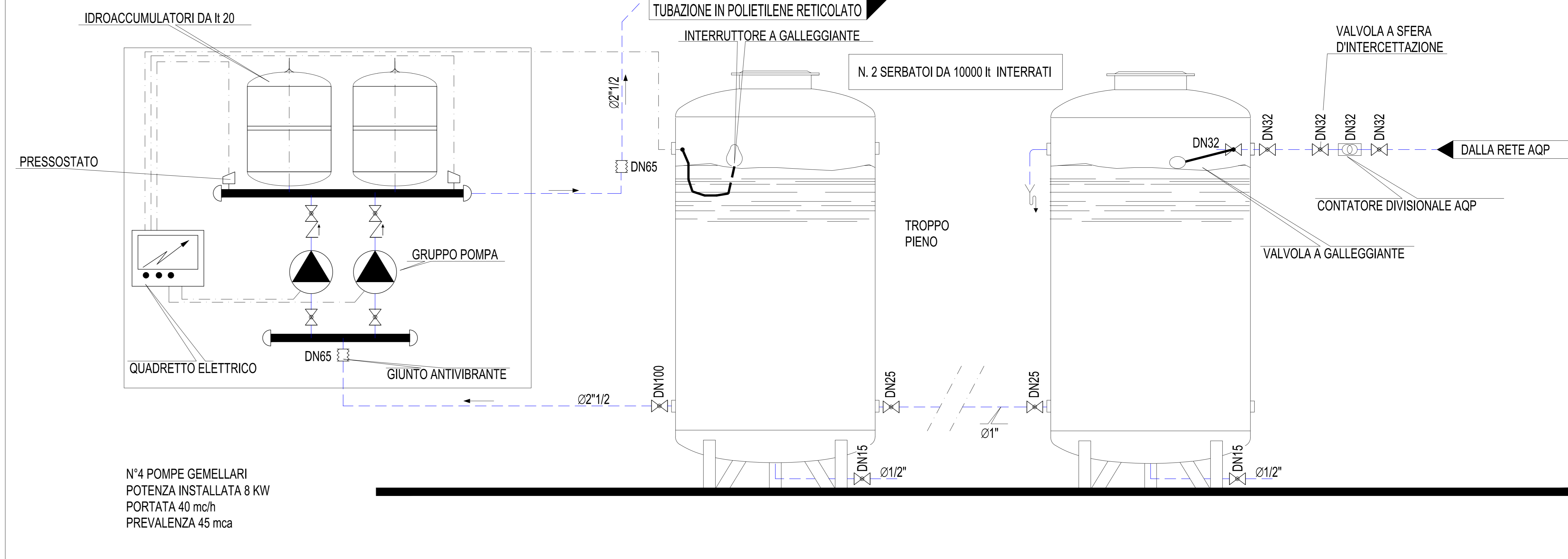
PARTICOLARI GRUPPO DI PRESSURIZZAZIONE IMPIANTO IDRICO ACQUA POTABILE
