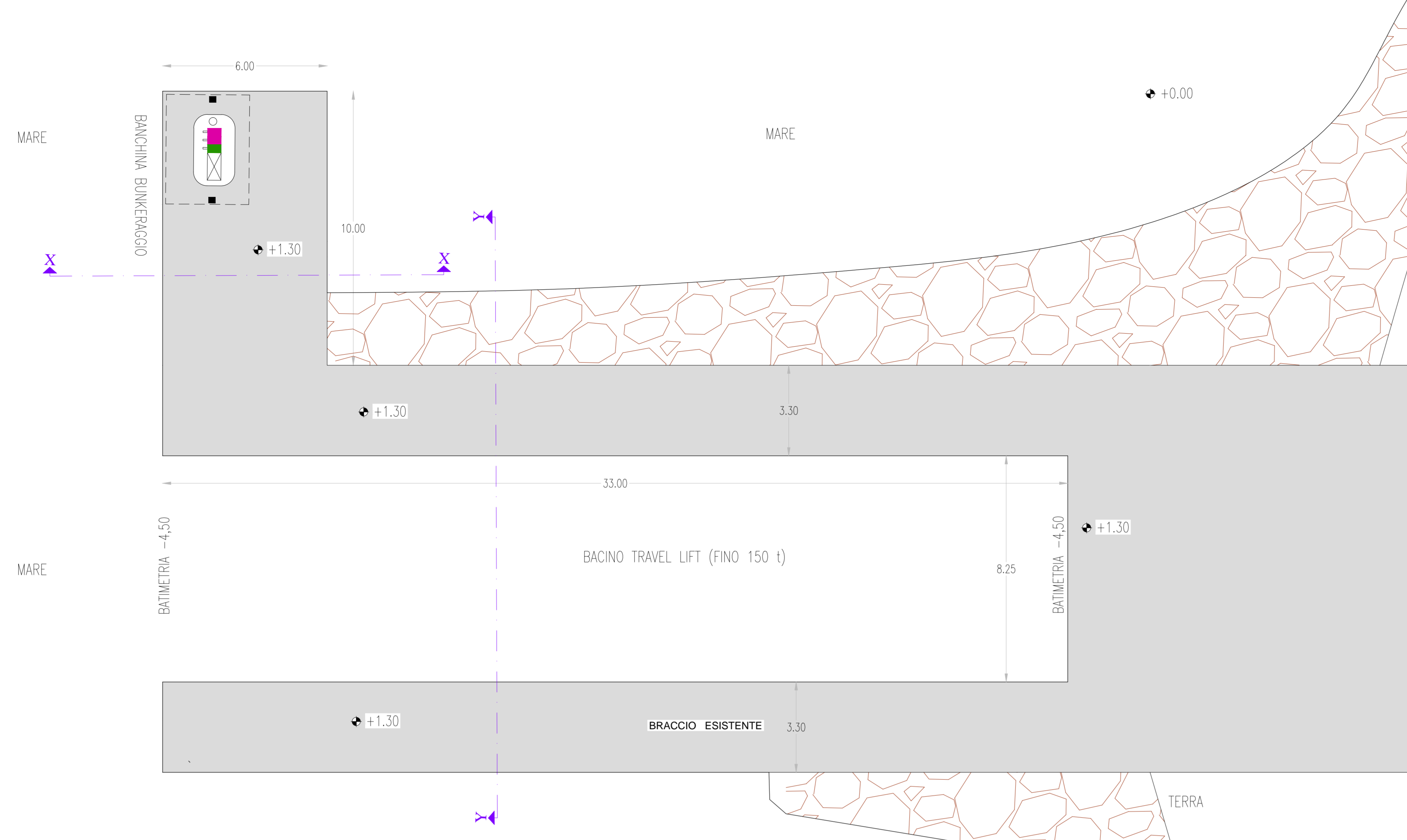
PROGETTO (PIANTA A QUOTA +2,00 m) 1:100
