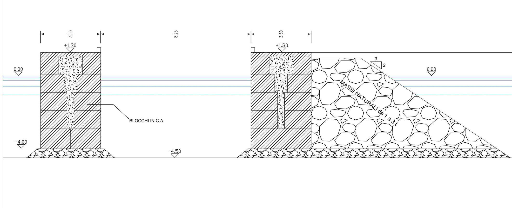
TRAVEL-LIFT - SEZIONE TRASVERSALE TIPO Y-Y 1:100
