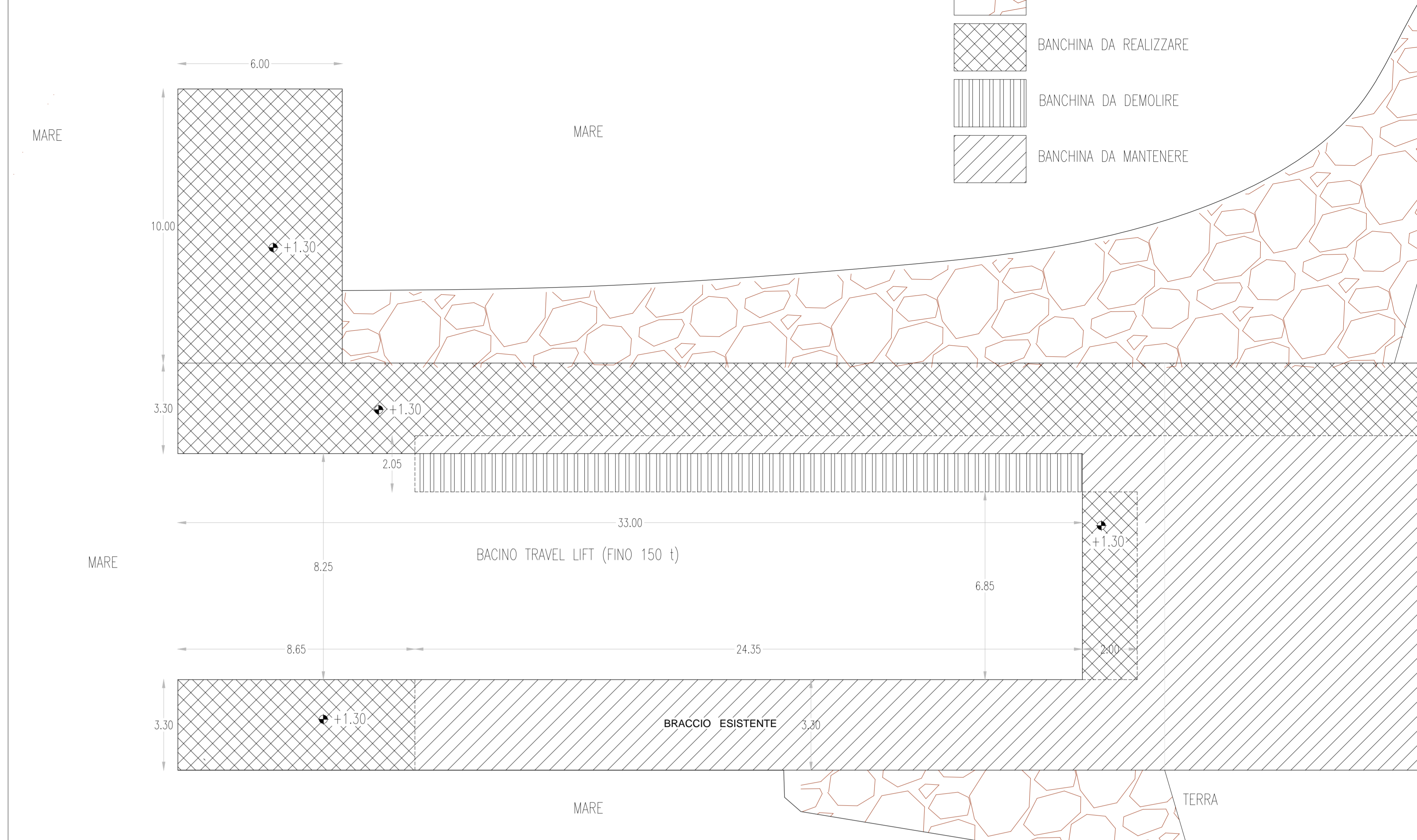
PIANO DEMOLIZIONI-COSTRUZIONI (PIANTA A QUOTA +2,00 m) 1:100
