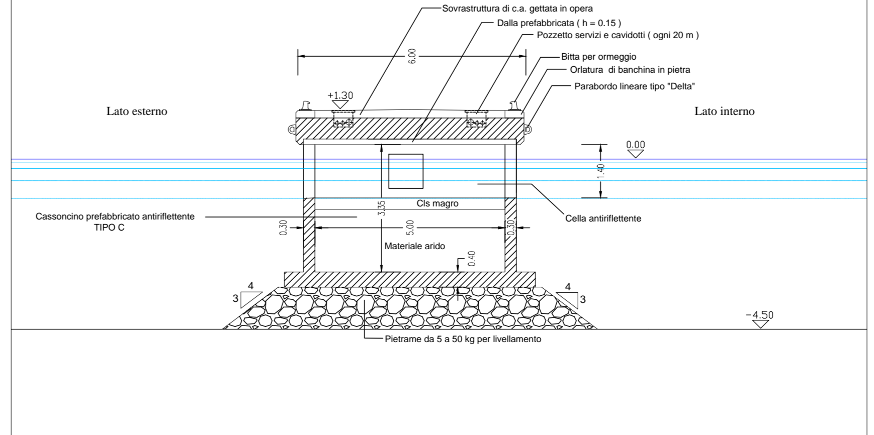
MOLO BUNKERAGGIO - SEZIONE TRASVERSALE TIPO X-X 1:100
