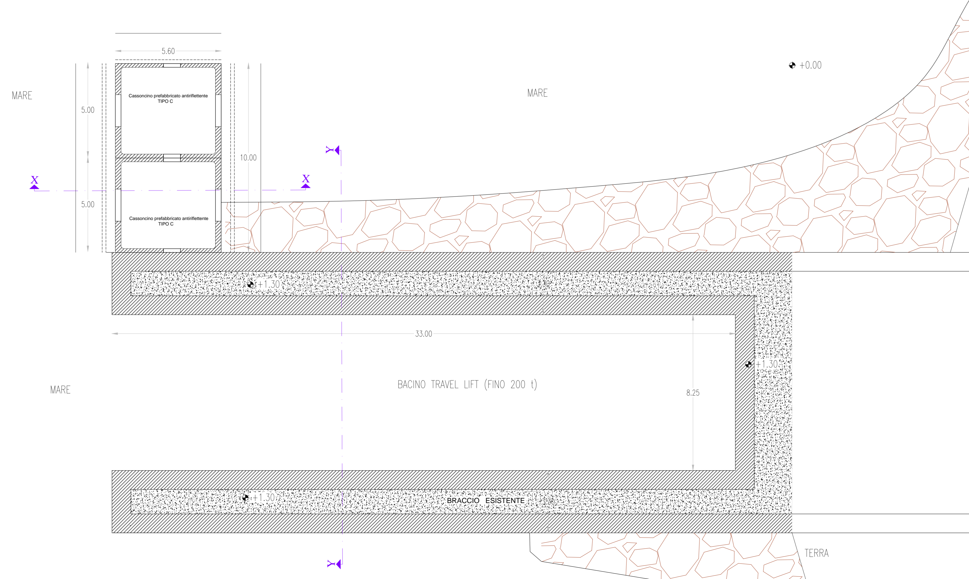
PROGETTO (PIANTA A QUOTA +0,5 m) 1:100
