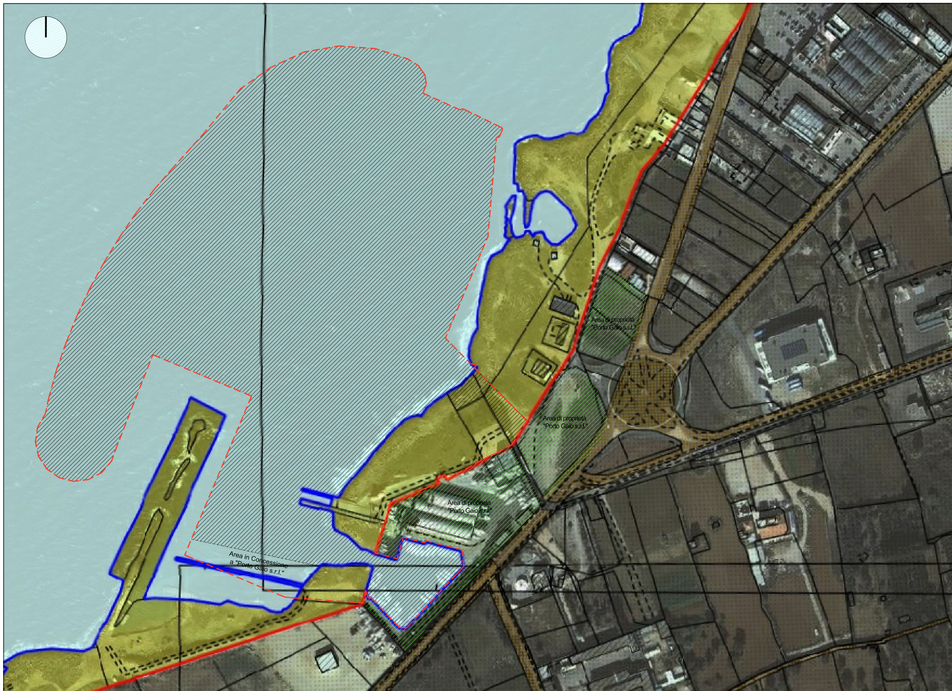
CARTOGRAFIA CATASTALE S.I.D. scala 1:2000
