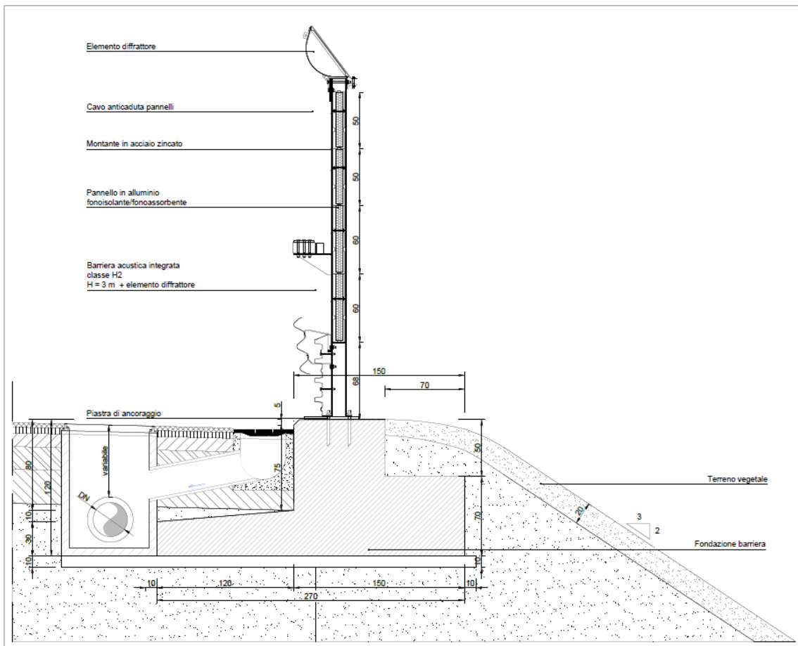
Figura 2.2.1 Sezione tipo barriera antirumore integrata su rilevato (Barriere n. 2 e 4)
