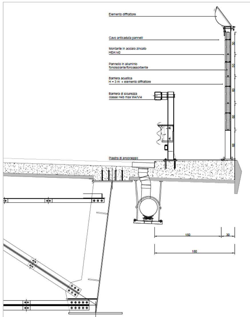
Figura 2.2.3 Sezione tipo barriera antirumore su viadotto nel tratto di superamento della ferrovia
