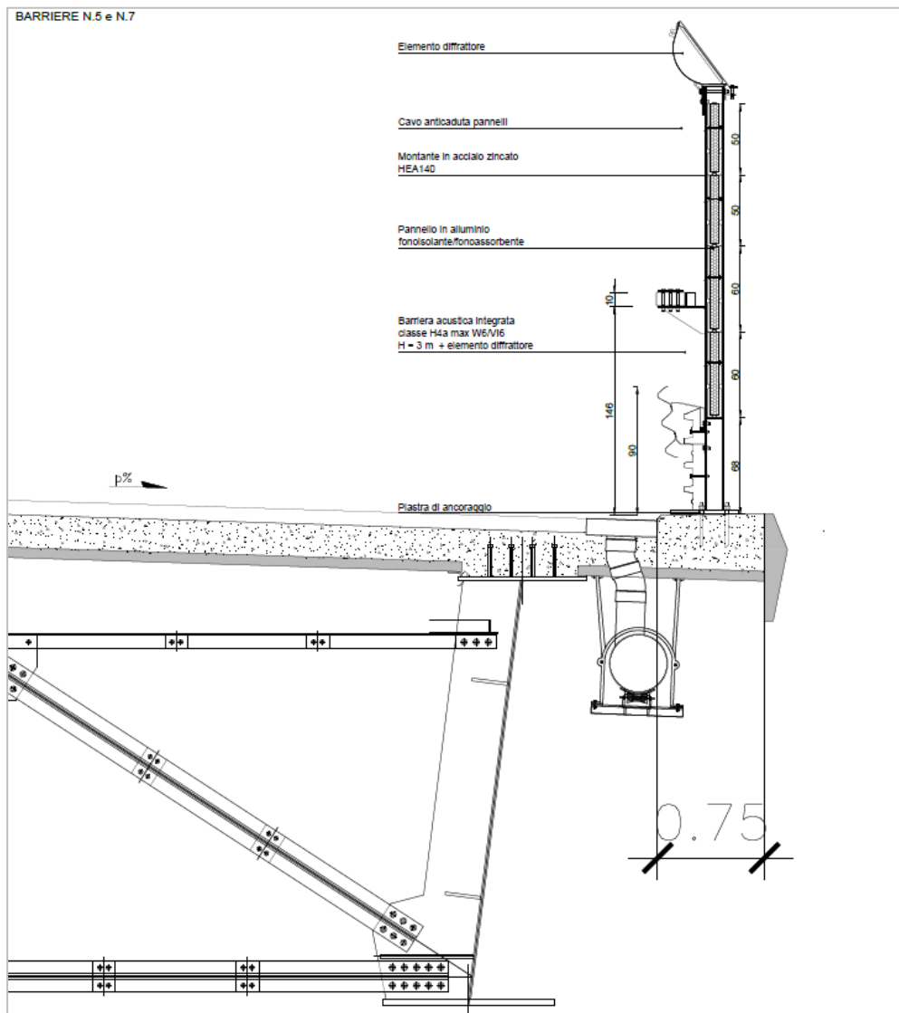
Figura 2.2.2 Sezione tipo barriera antirumore integrata su viadotto (Barriere 5 e 7)
