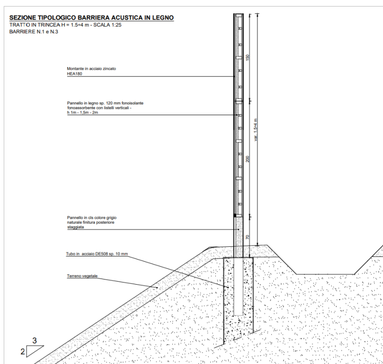
Figura 2.1.1 Sezione tipo barriera antirumore in legno
